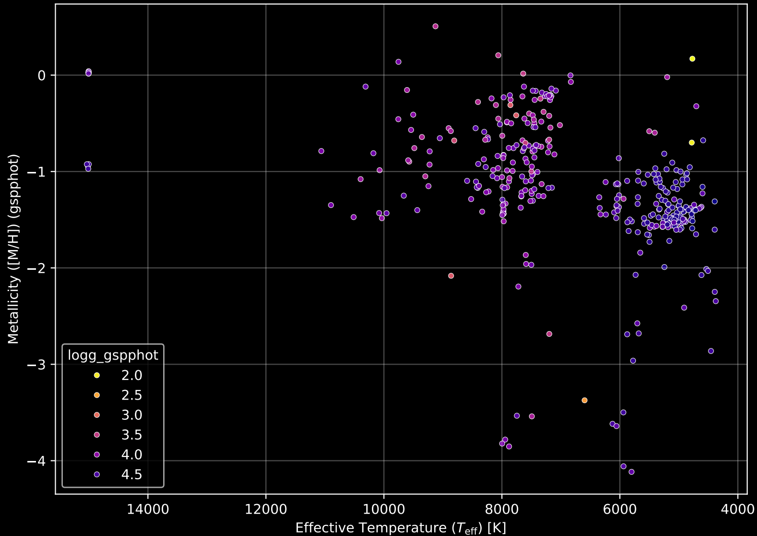
Gaia Cluster: [NGC_6192] Stellar Population Parameters (n= 373)
