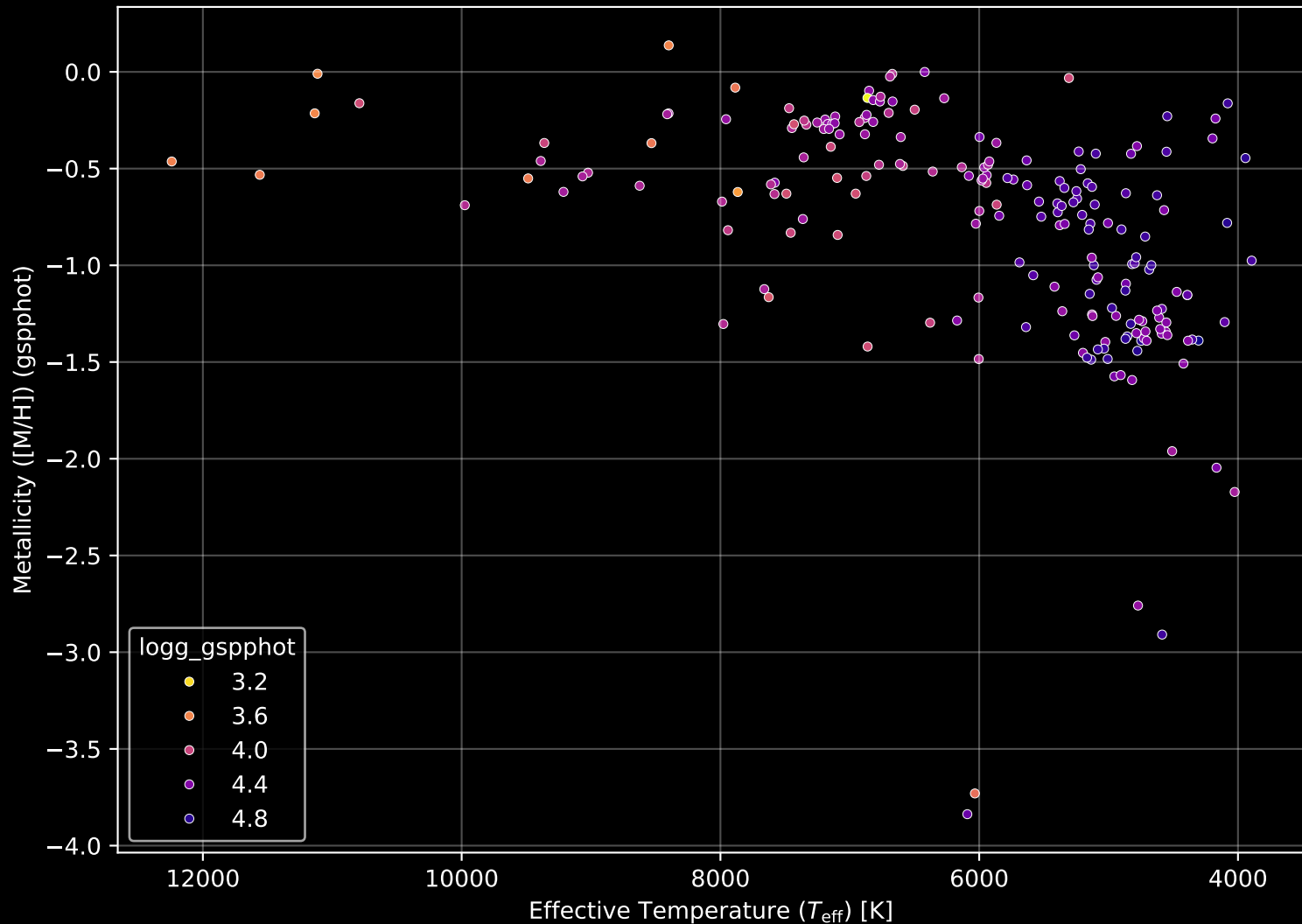
Gaia Cluster: [NGC_6204] Stellar Population Parameters (n= 201)
