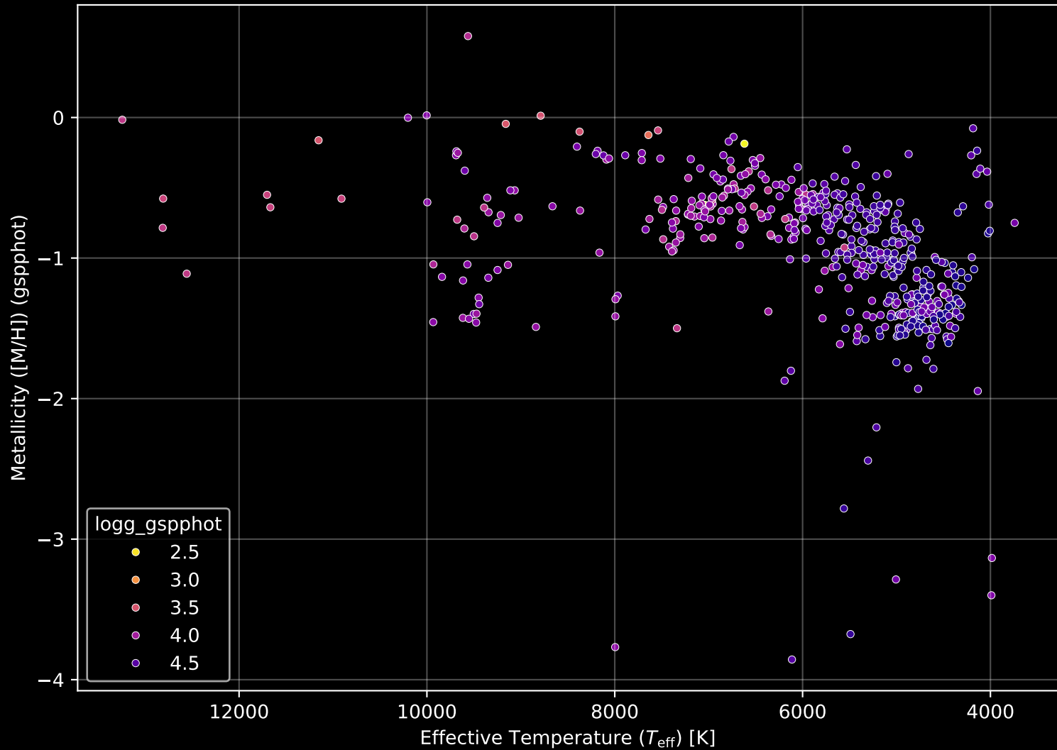
Gaia Cluster: [NGC_6242] Stellar Population Parameters (n= 523)
