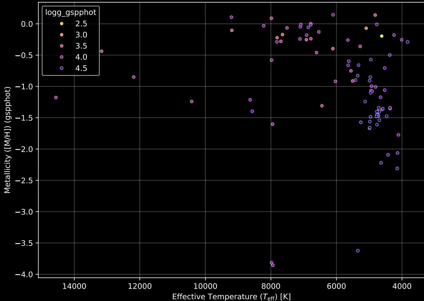
Gaia Cluster: [NGC_6322] Stellar Population Parameters (n= 89)
