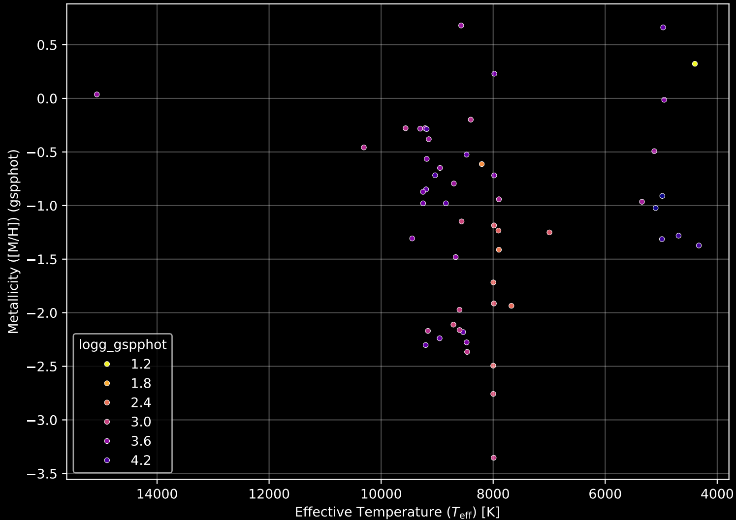
Gaia Cluster: [NGC_6357] Stellar Population Parameters (n= 54)
