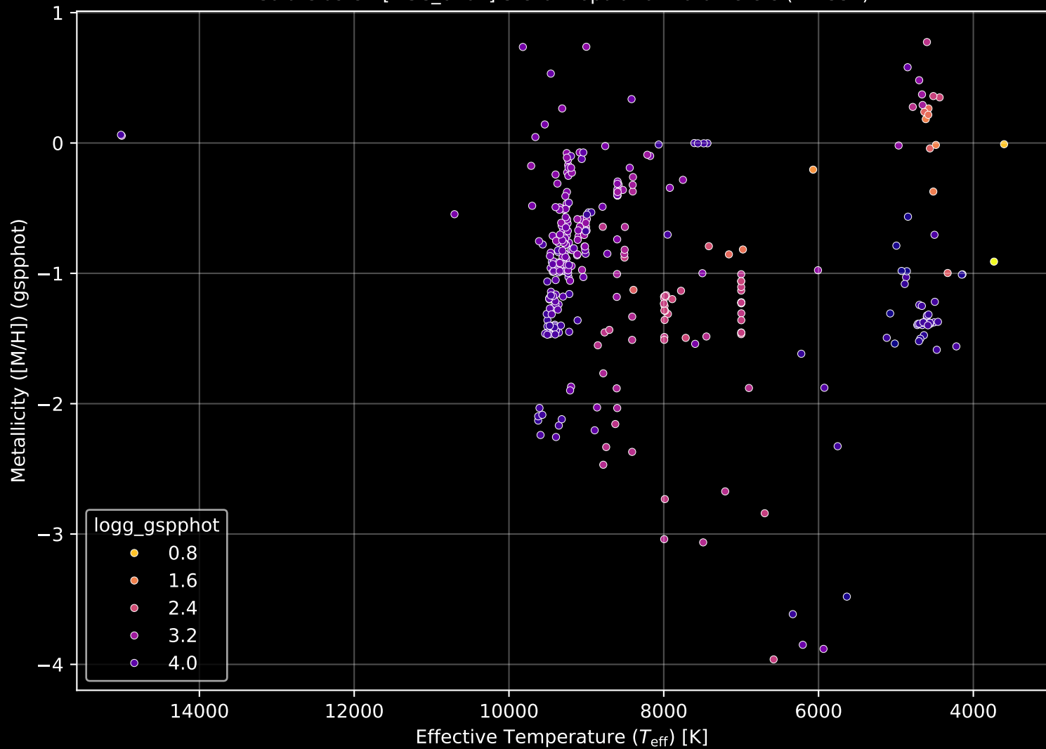
Gaia Cluster: [NGC_6404] Stellar Population Parameters (n= 334)
