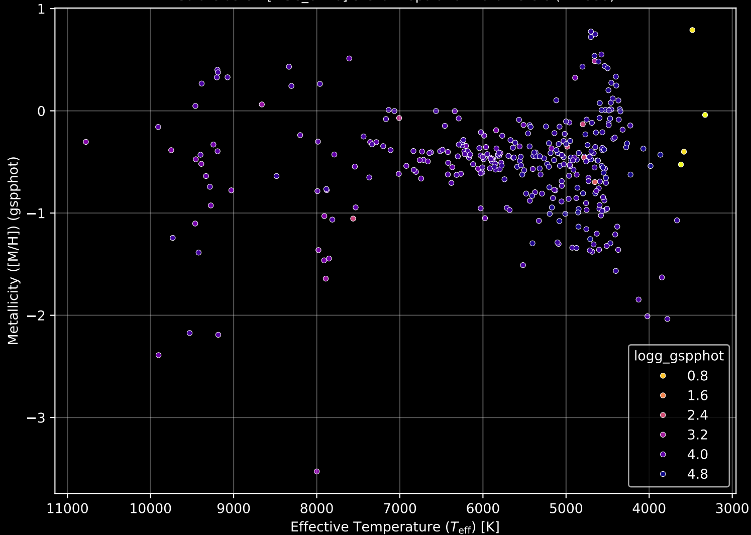
Gaia Cluster: [NGC_6416] Stellar Population Parameters (n= 333)
