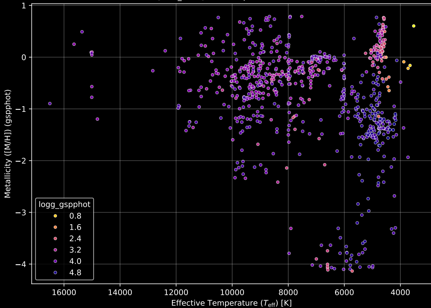
Gaia Cluster: [NGC_6451] Stellar Population Parameters (n= 752)
