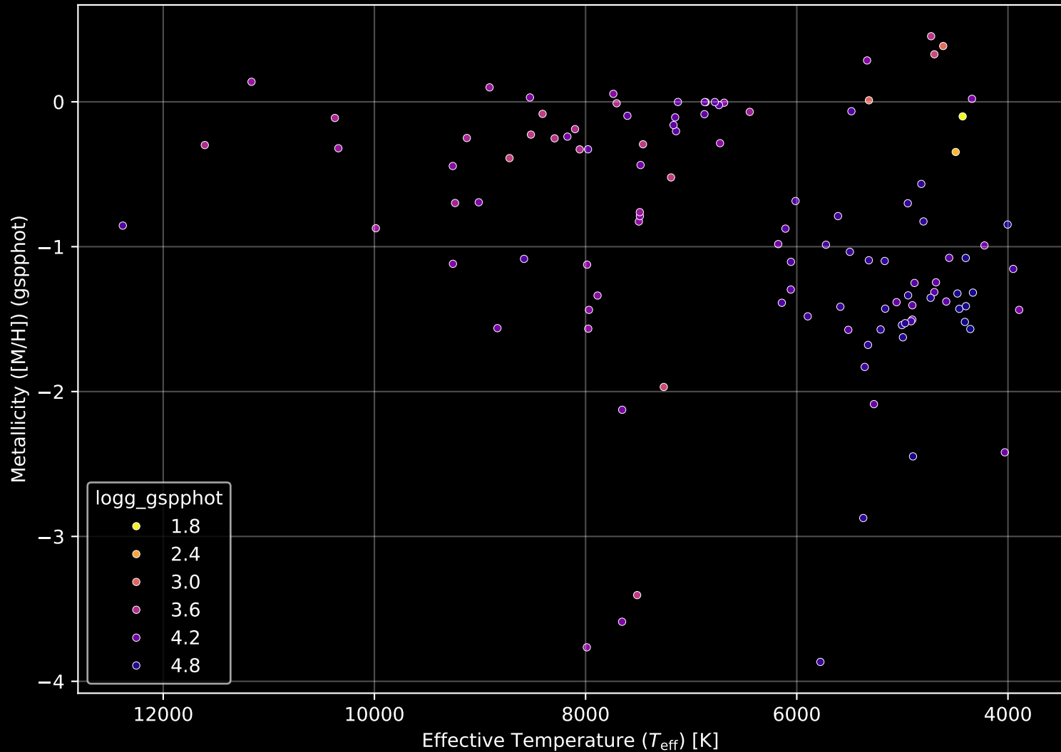
Gaia Cluster: [NGC_6469] Stellar Population Parameters (n= 113)
