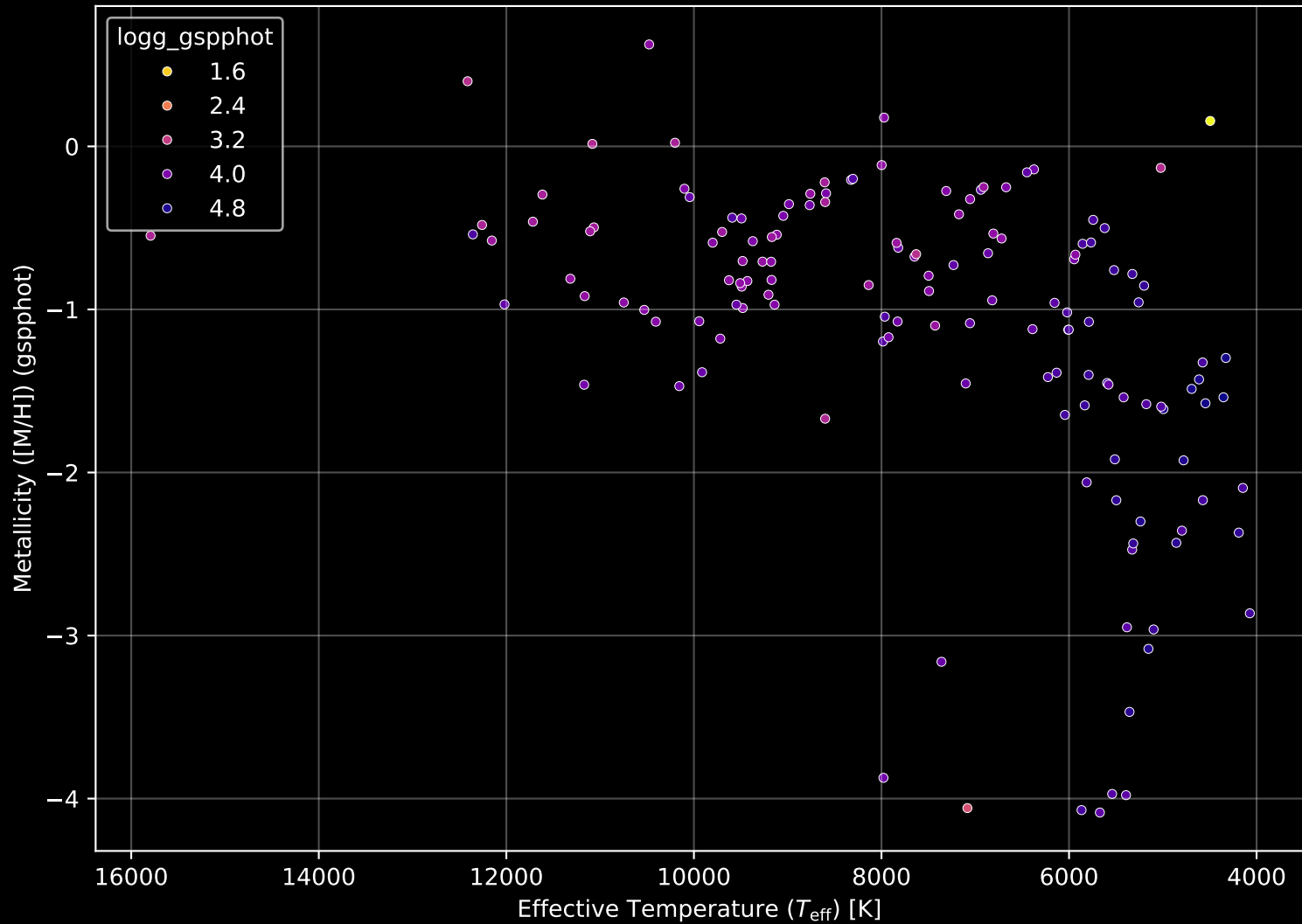
Gaia Cluster: [NGC_6520] Stellar Population Parameters (n= 142)
