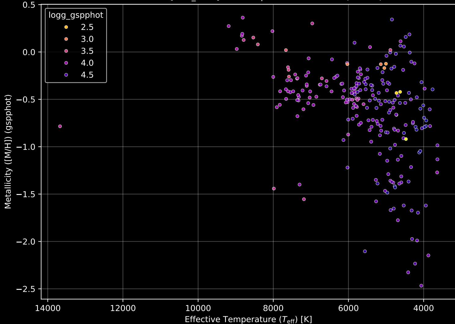
Gaia Cluster: [NGC_6568] Stellar Population Parameters (n= 243)
