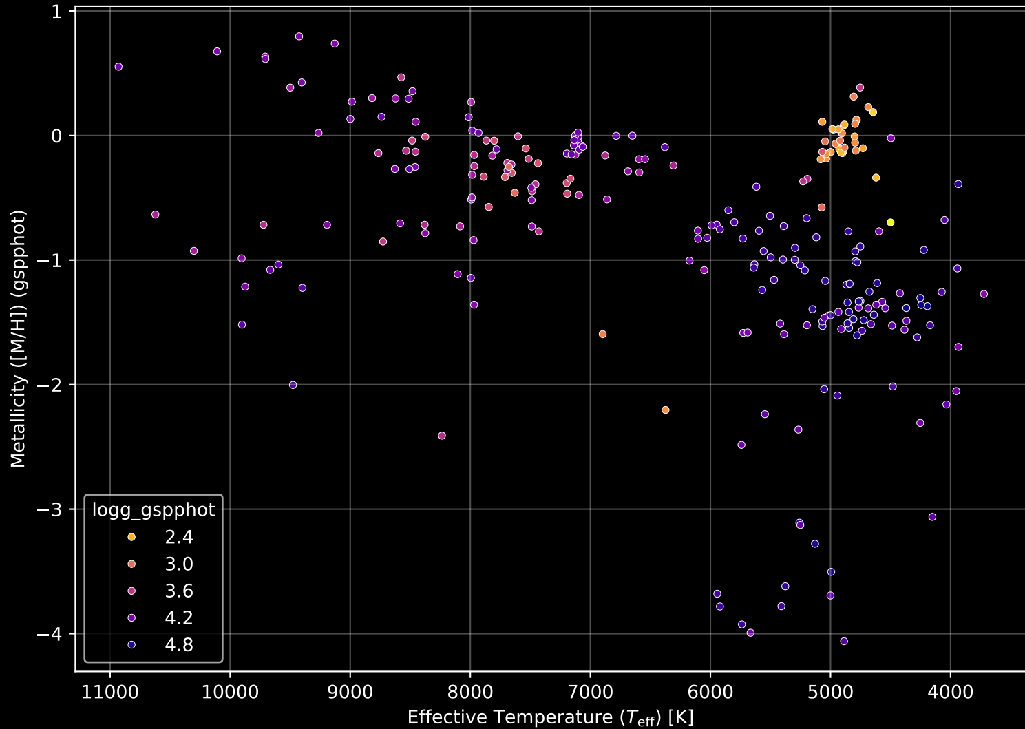
Gaia Cluster: [NGC_6583] Stellar Population Parameters (n= 255)
