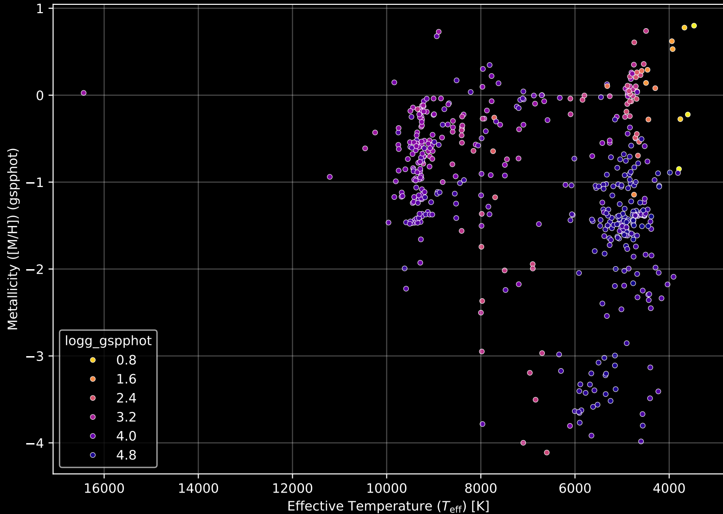
Gaia Cluster: [NGC_6631] Stellar Population Parameters (n= 512)
