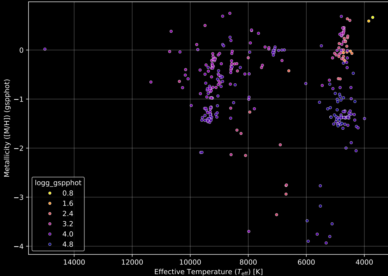
Gaia Cluster: [NGC_6756] Stellar Population Parameters (n= 306)
