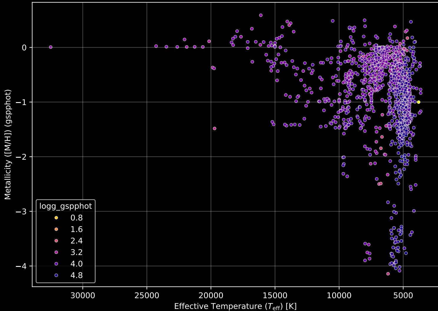
Gaia Cluster: [NGC_6871] Stellar Population Parameters (n= 1497)
