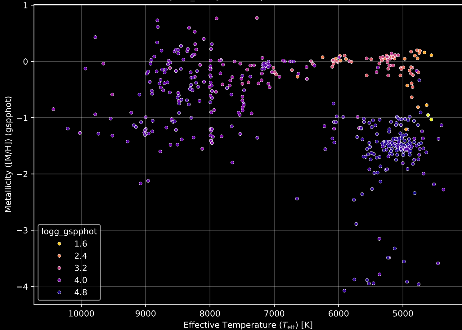
Gaia Cluster: [NGC_7044] Stellar Population Parameters (n= 515)
