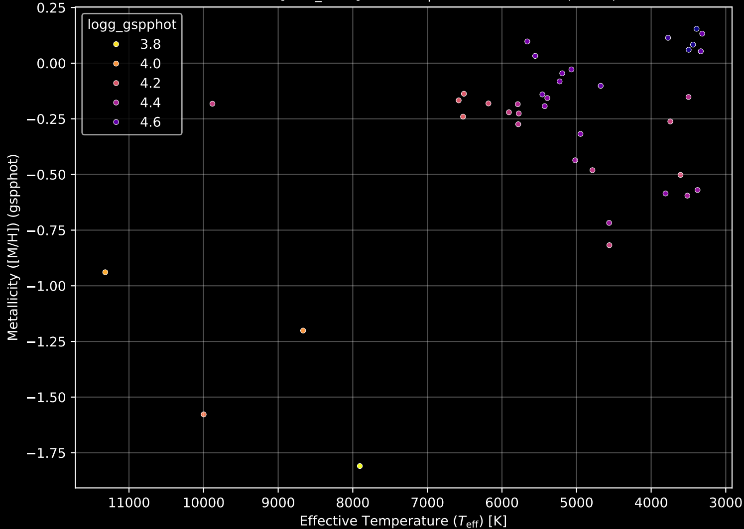
Gaia Cluster: [NGC_7058] Stellar Population Parameters (n= 39)
