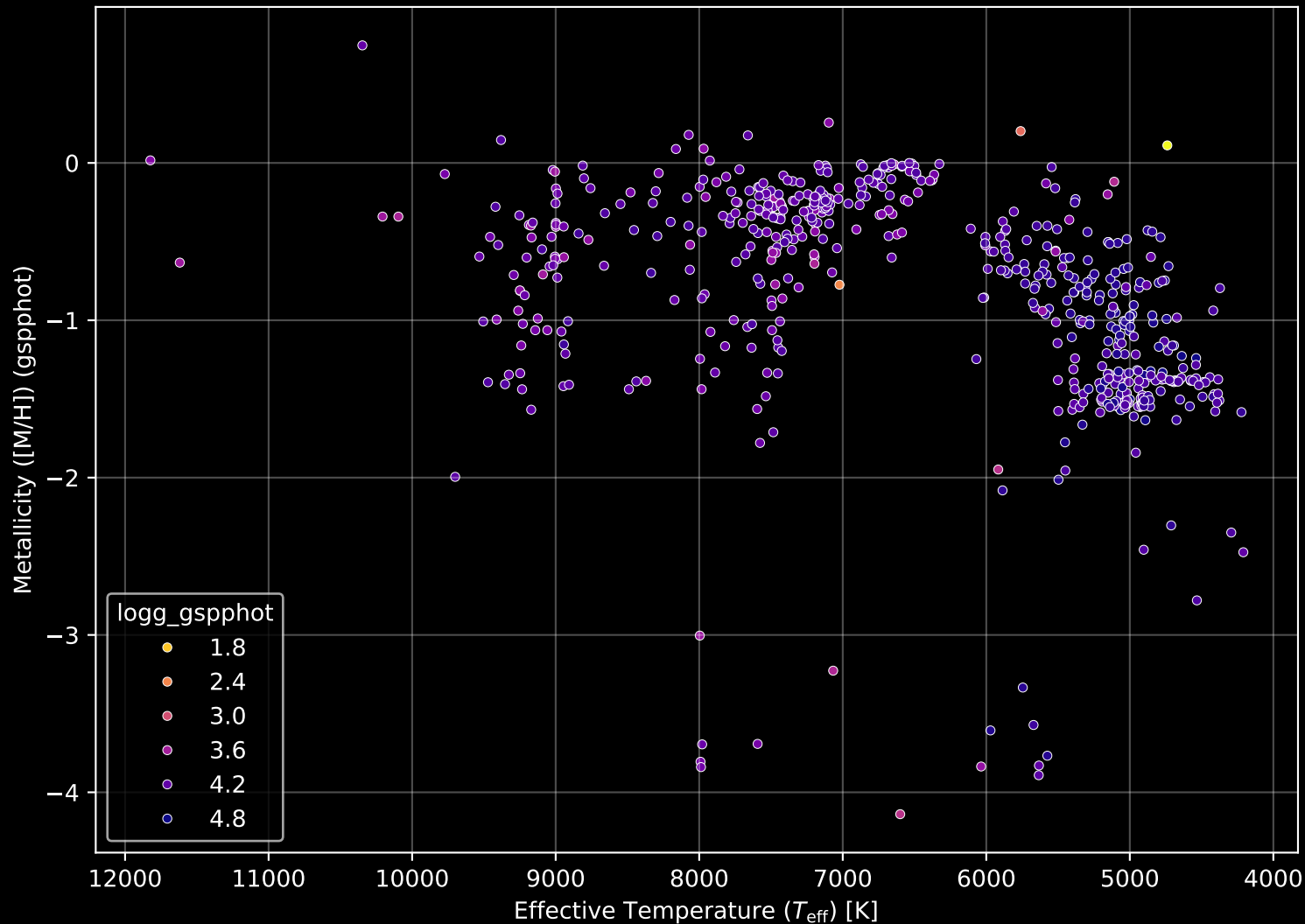
Gaia Cluster: [NGC_7086] Stellar Population Parameters (n= 602)
