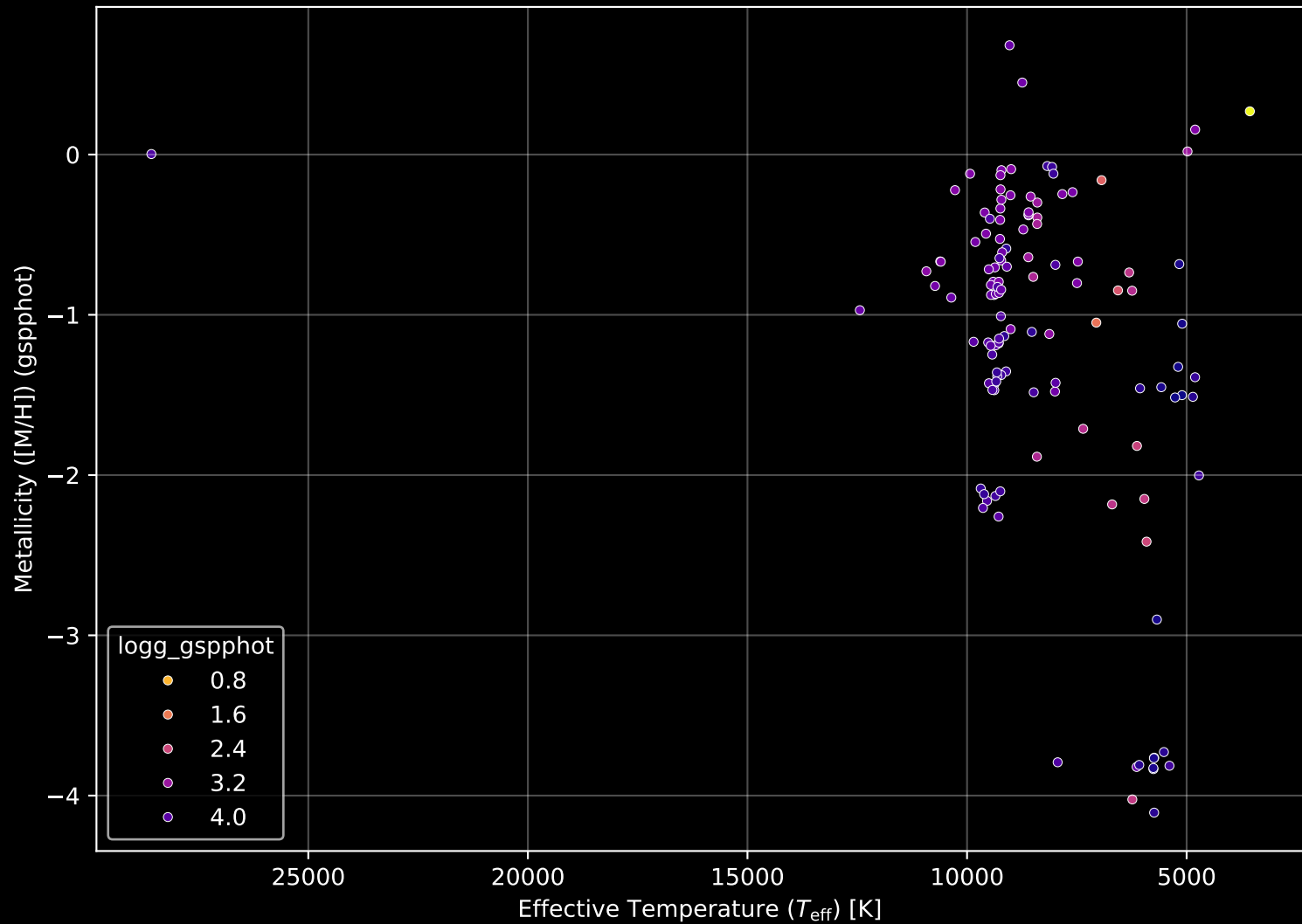
Gaia Cluster: [NGC_7128] Stellar Population Parameters (n= 126)
