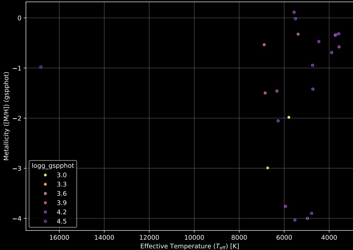
Gaia Cluster: [NGC 7129] Stellar Population Parameters (n= 22)
