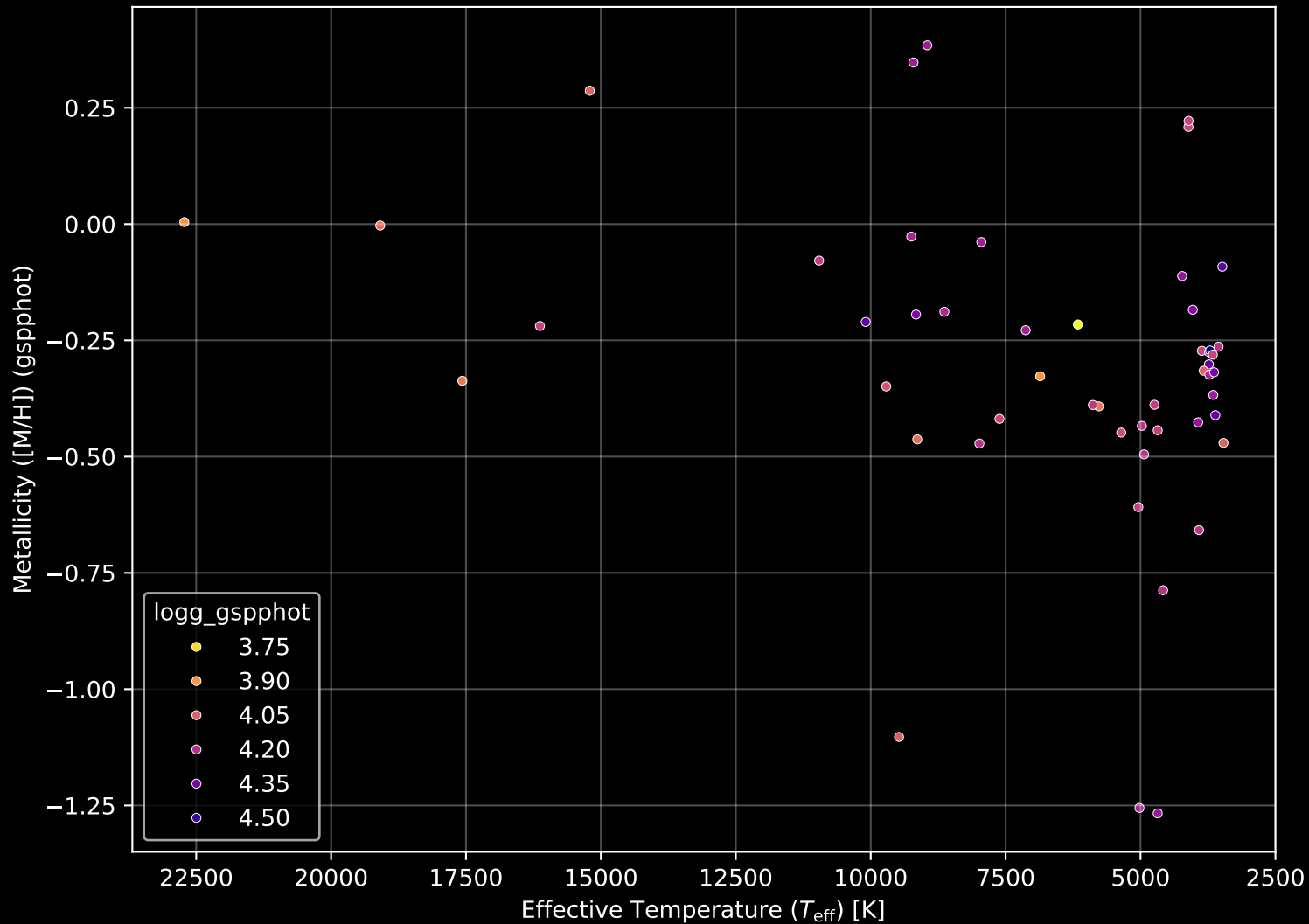
Gaia Cluster: [NGC_7160] Stellar Population Parameters (n= 51)
