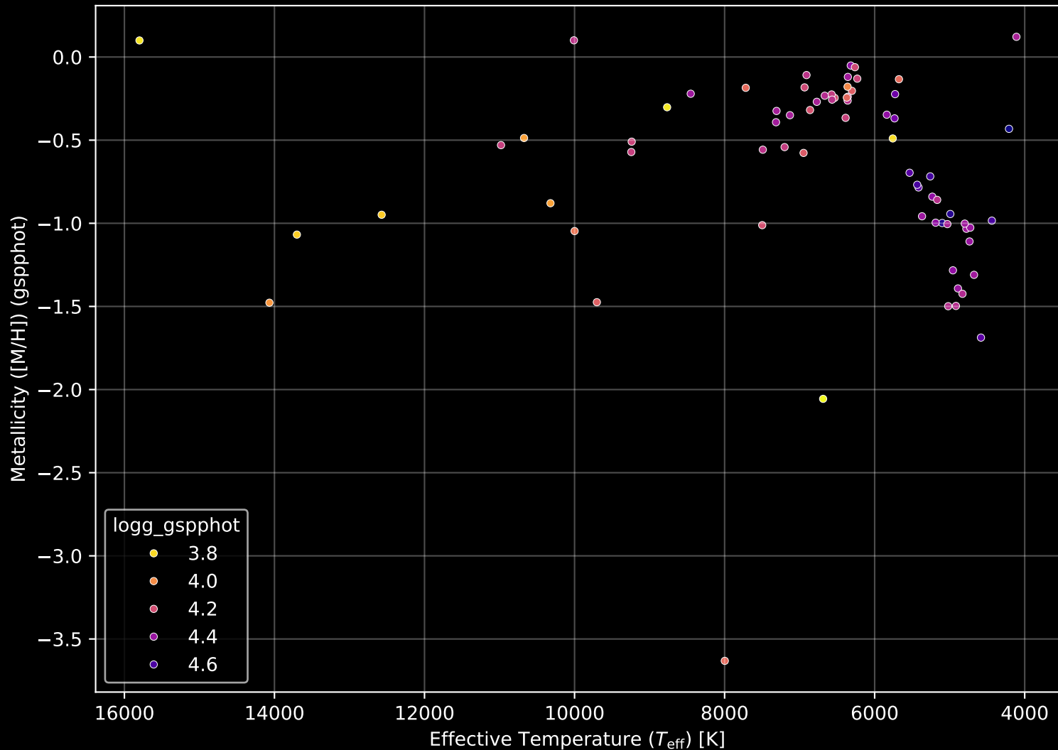
Gaia Cluster: [NGC_743] Stellar Population Parameters (n= 72)
