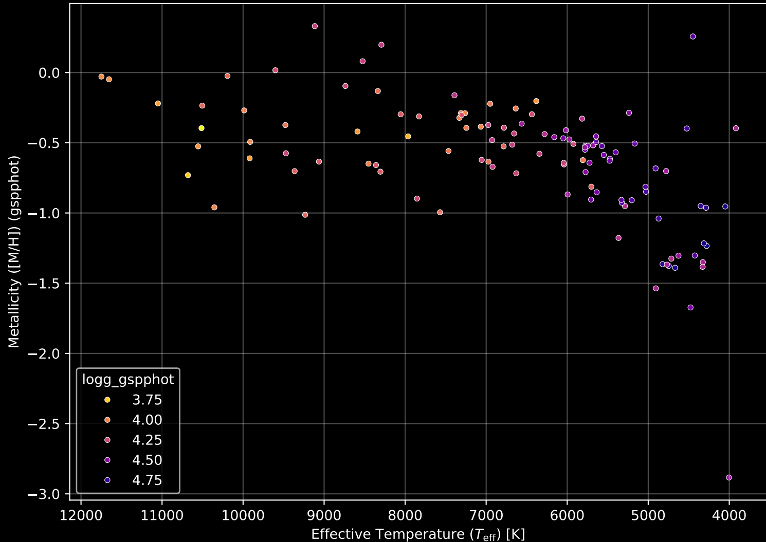
Gaia Cluster: [NGC_744] Stellar Population Parameters (n= 116)
