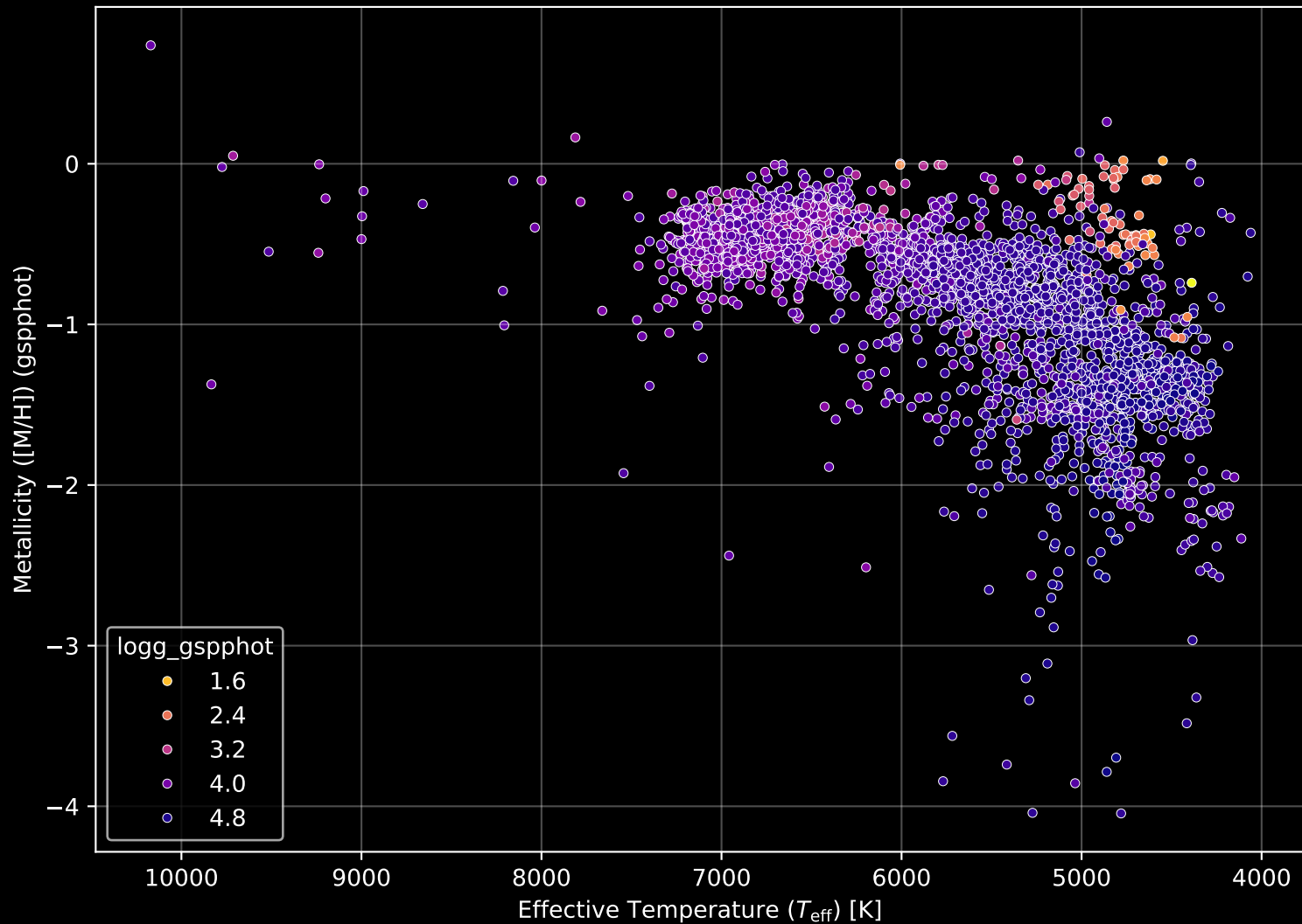
Gaia Cluster: [NGC_7789] Stellar Population Parameters (n= 3347)
