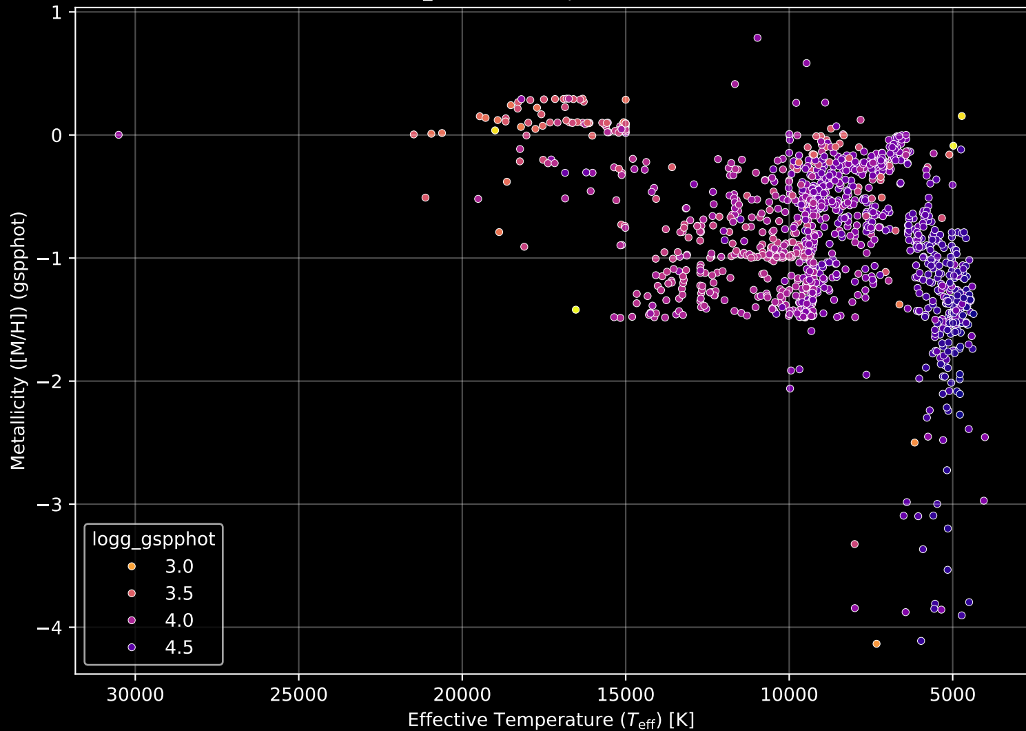
Gaia Cluster: [NGC_869] Stellar Population Parameters (n= 1262)
