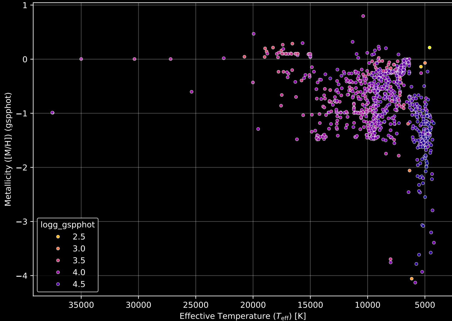
Gaia Cluster: [NGC_884] Stellar Population Parameters (n= 981)
