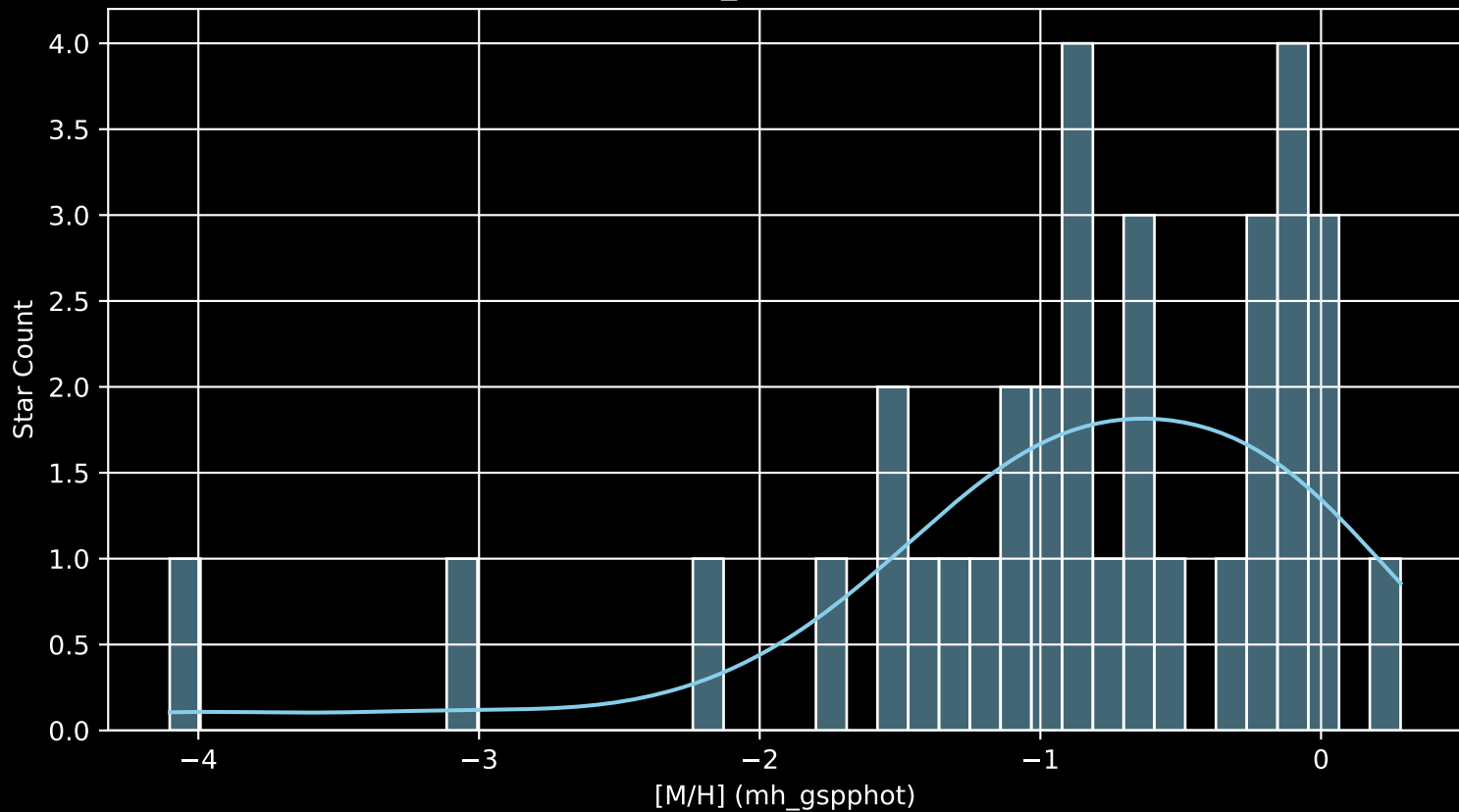
Gaia Cluster: [Pismis_11 [M/H] (mh_gspphot) (n= 34)
