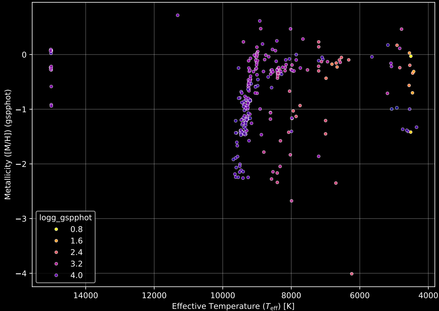
Gaia Cluster: [Pismis_19] Stellar Population Parameters (n= 283)
