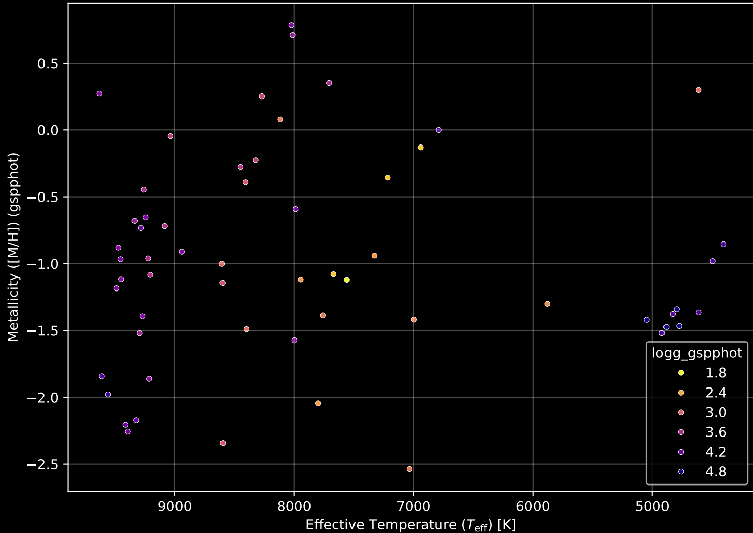
Gaia Cluster: [Pismis_23] Stellar Population Parameters (n= 58)
