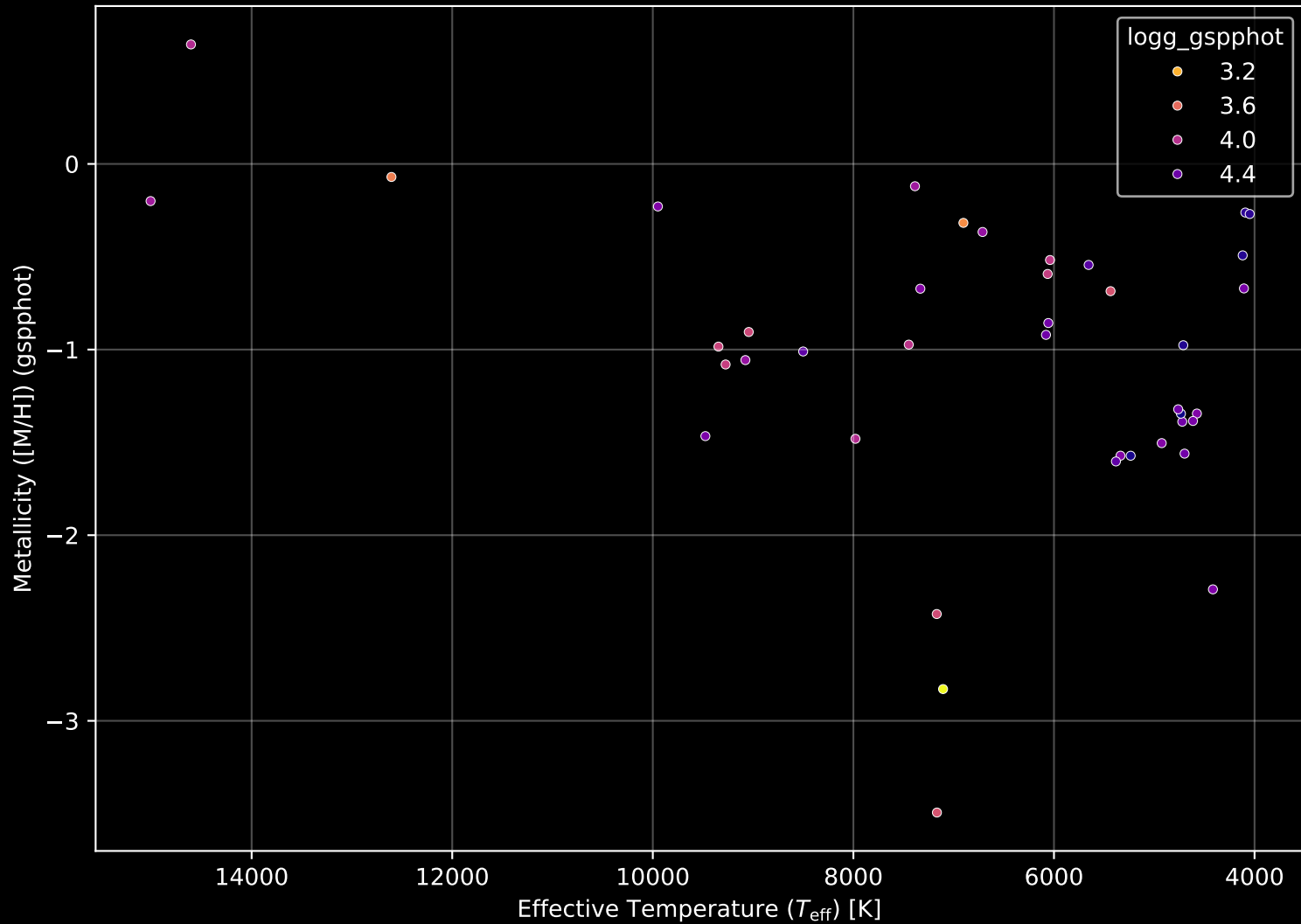
Gaia Cluster: [Pismis_27] Stellar Population Parameters (n= 41)
