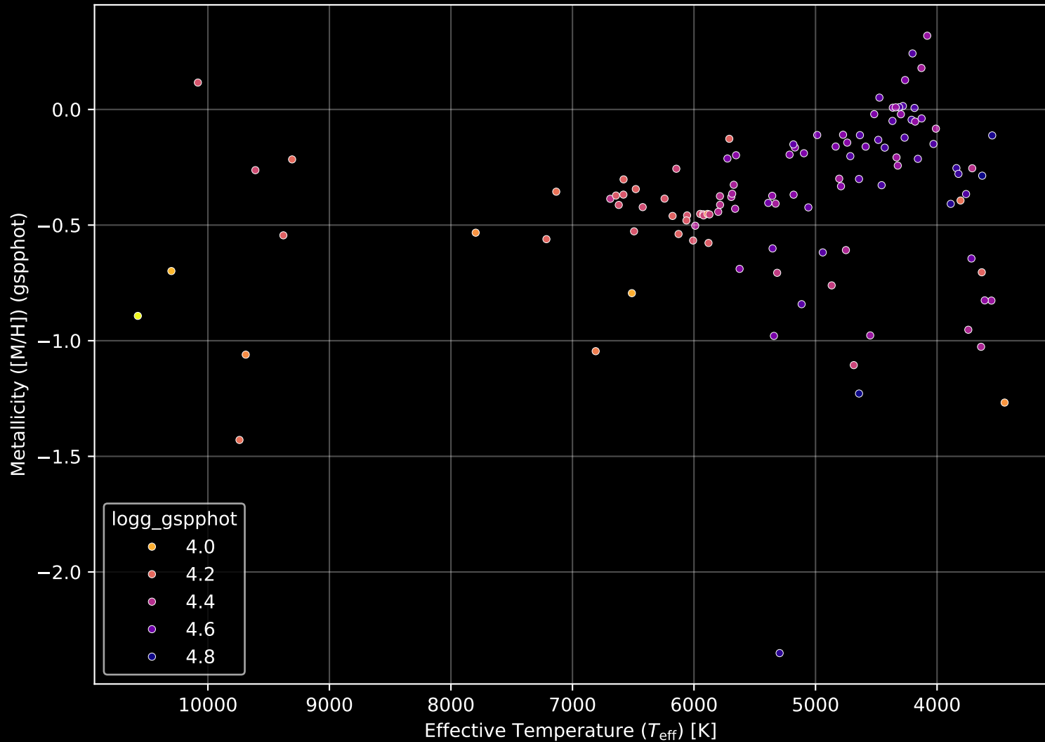
Gaia Cluster: [Pismis_4] Stellar Population Parameters (n= 116)
