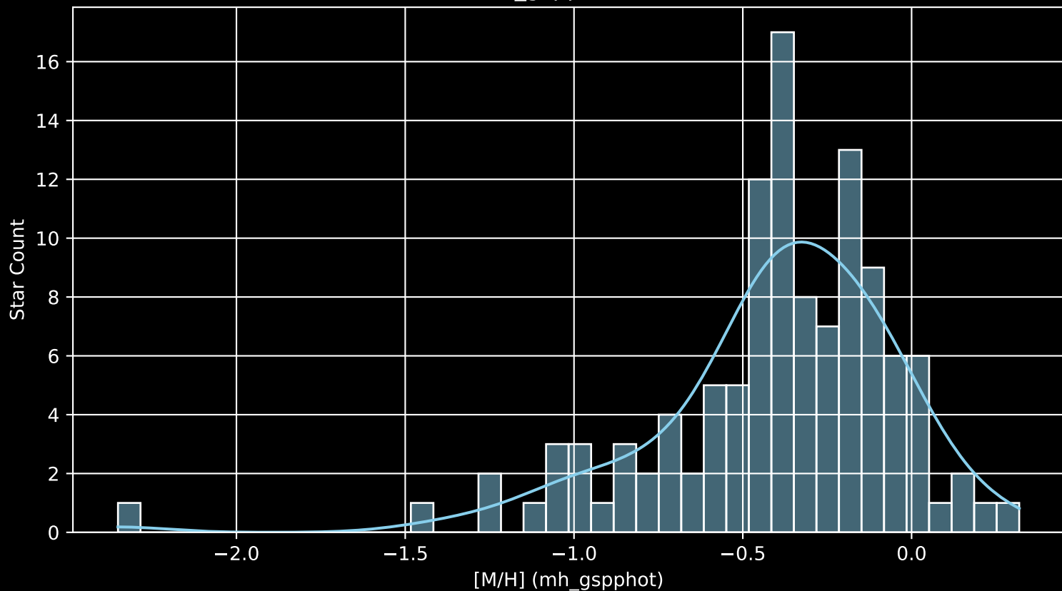
Gaia Cluster: [Pismis_4 [M/H] (mh_gspphot) (n= 116)
