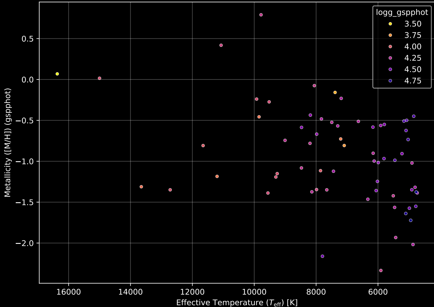
Gaia Cluster: [Pismis_8] Stellar Population Parameters (n= 66)
