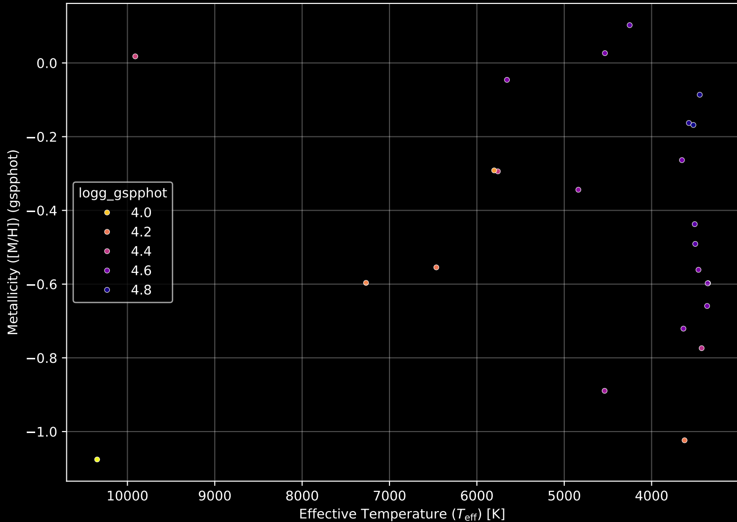
Gaia Cluster: [Platais_10] Stellar Population Parameters (n= 24)
