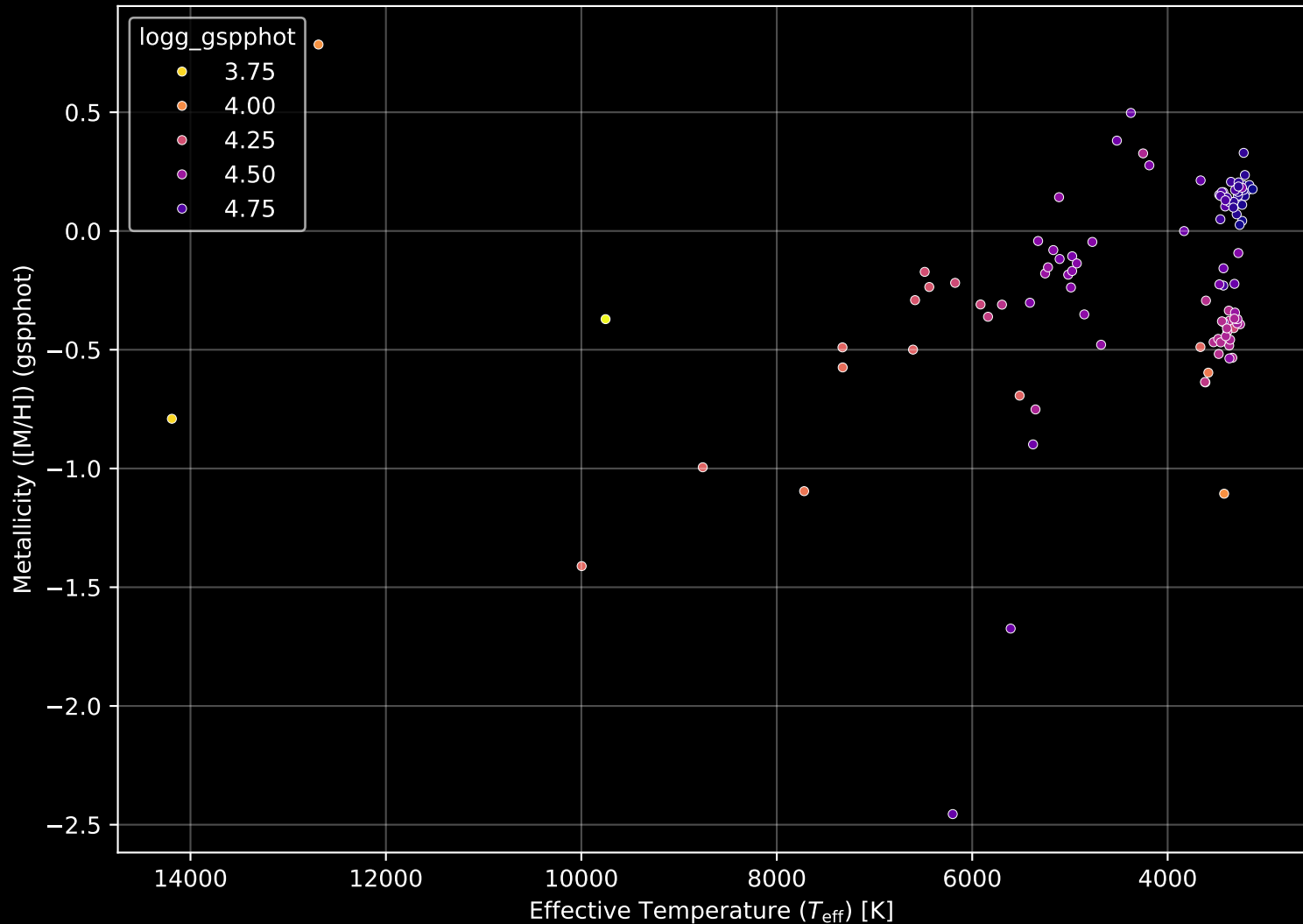
Gaia Cluster: [Platais_9] Stellar Population Parameters (n= 116)
