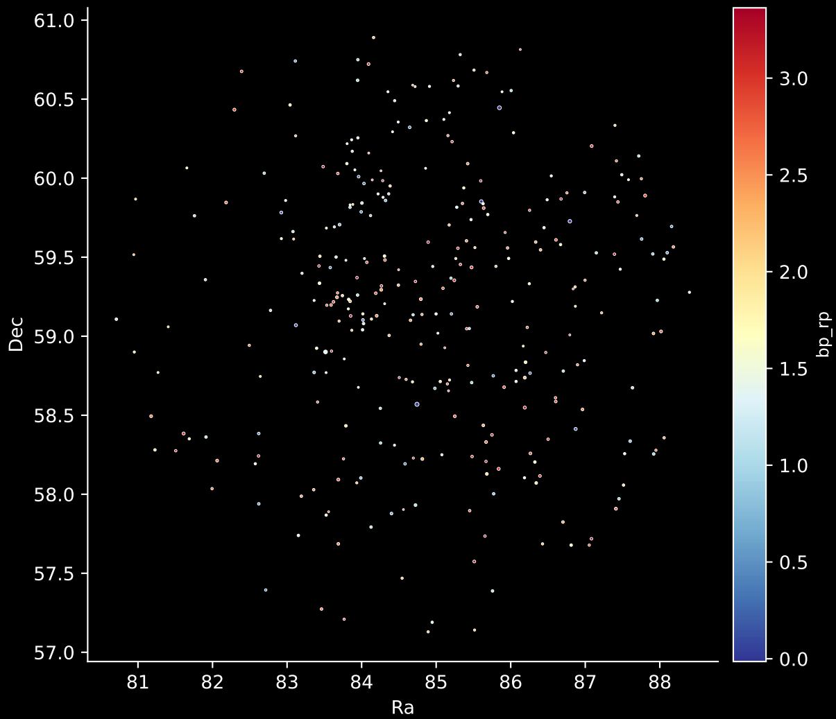
Gaia Cluster: [RSG_8] Stars: 316
