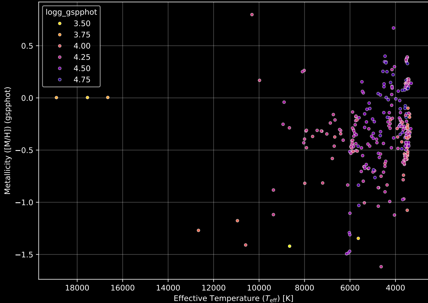
Gaia Cluster: [RSG_8] Stellar Population Parameters (n= 316)
