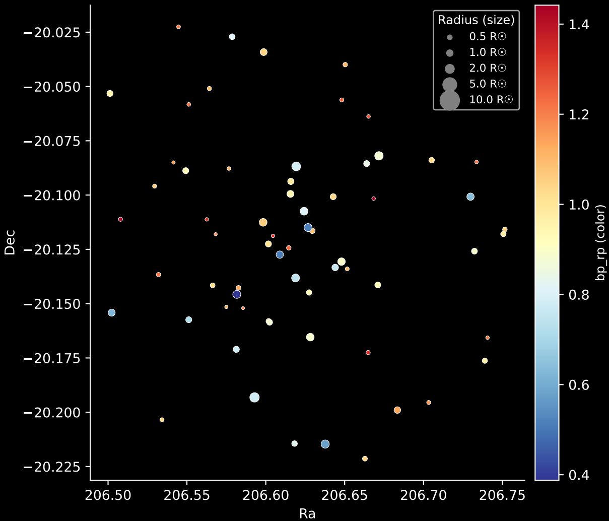
Gaia Cluster: [Ruprecht_10] Stars: 65
