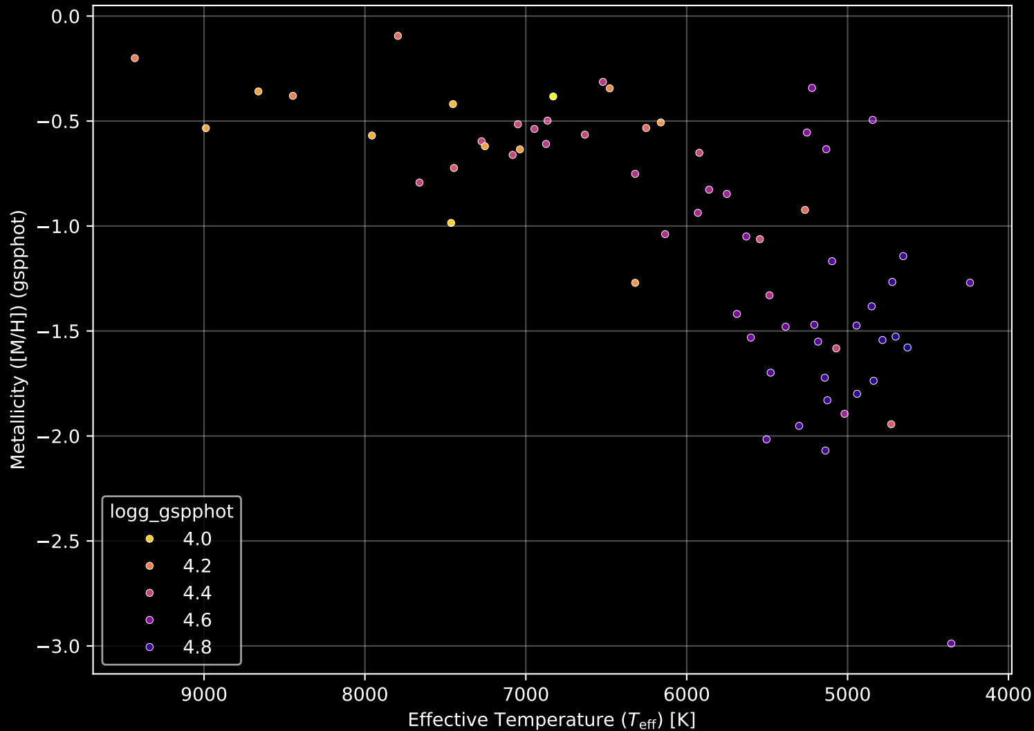
Gaia Cluster: [Ruprecht_10] Stellar Population Parameters (n= 65)
