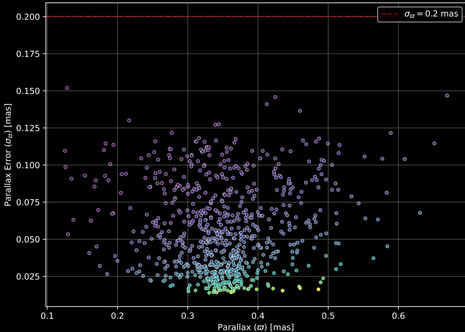
Gaia Cluster: [Ruprecht_112] Parallax Quality (n= 740)
