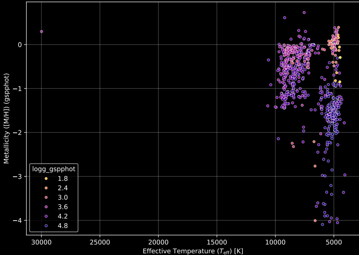
Gaia Cluster: [Ruprecht_112] Stellar Population Parameters (n= 740)
