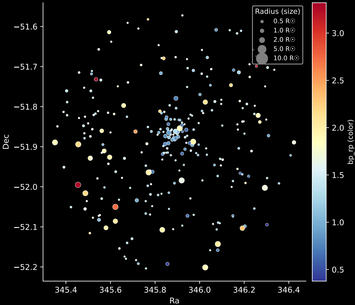
Gaia Cluster: [Ruprecht_117] Stars: 272
