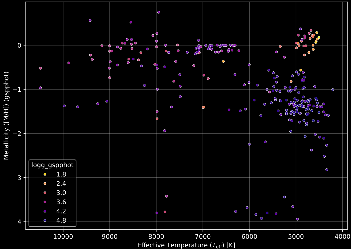
Gaia Cluster: [Ruprecht_117] Stellar Population Parameters (n= 272)
