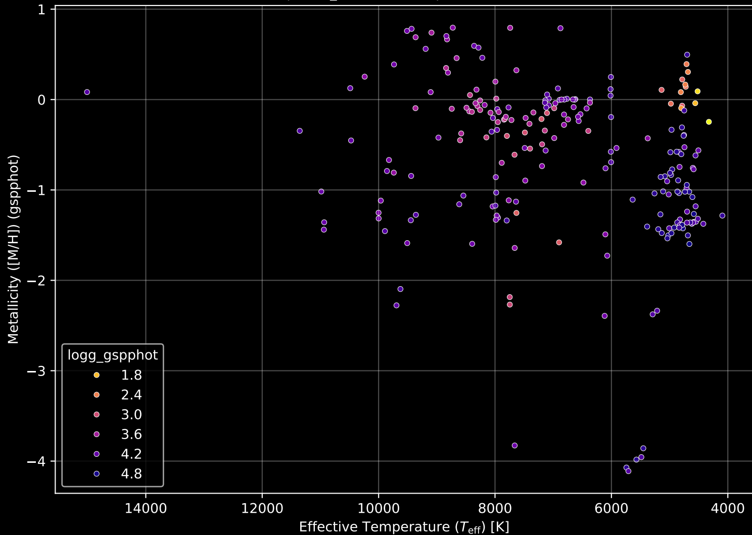
Gaia Cluster: [Ruprecht_128] Stellar Population Parameters (n= 229)
