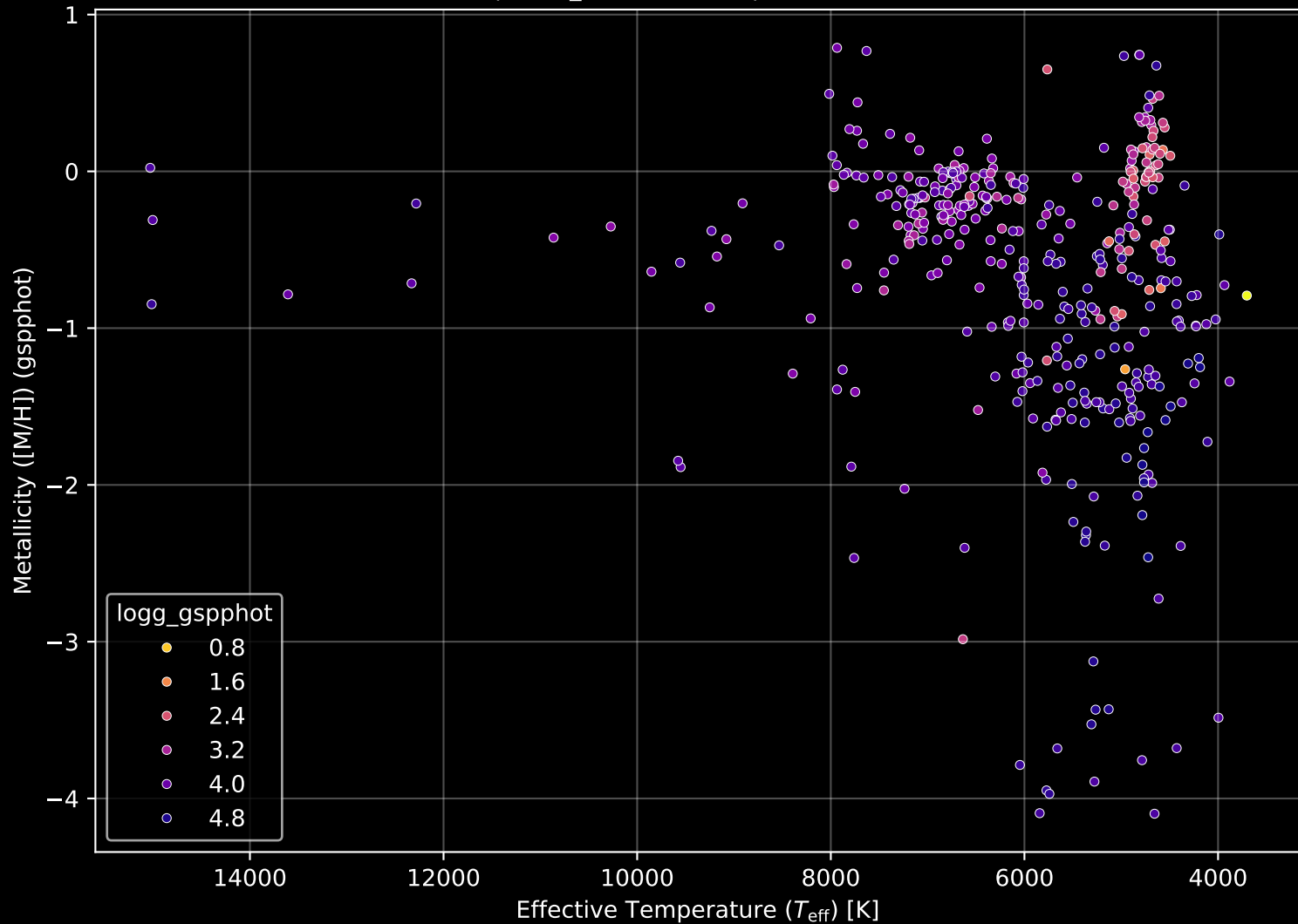
Gaia Cluster: [Ruprecht_134] Stellar Population Parameters (n= 413)
