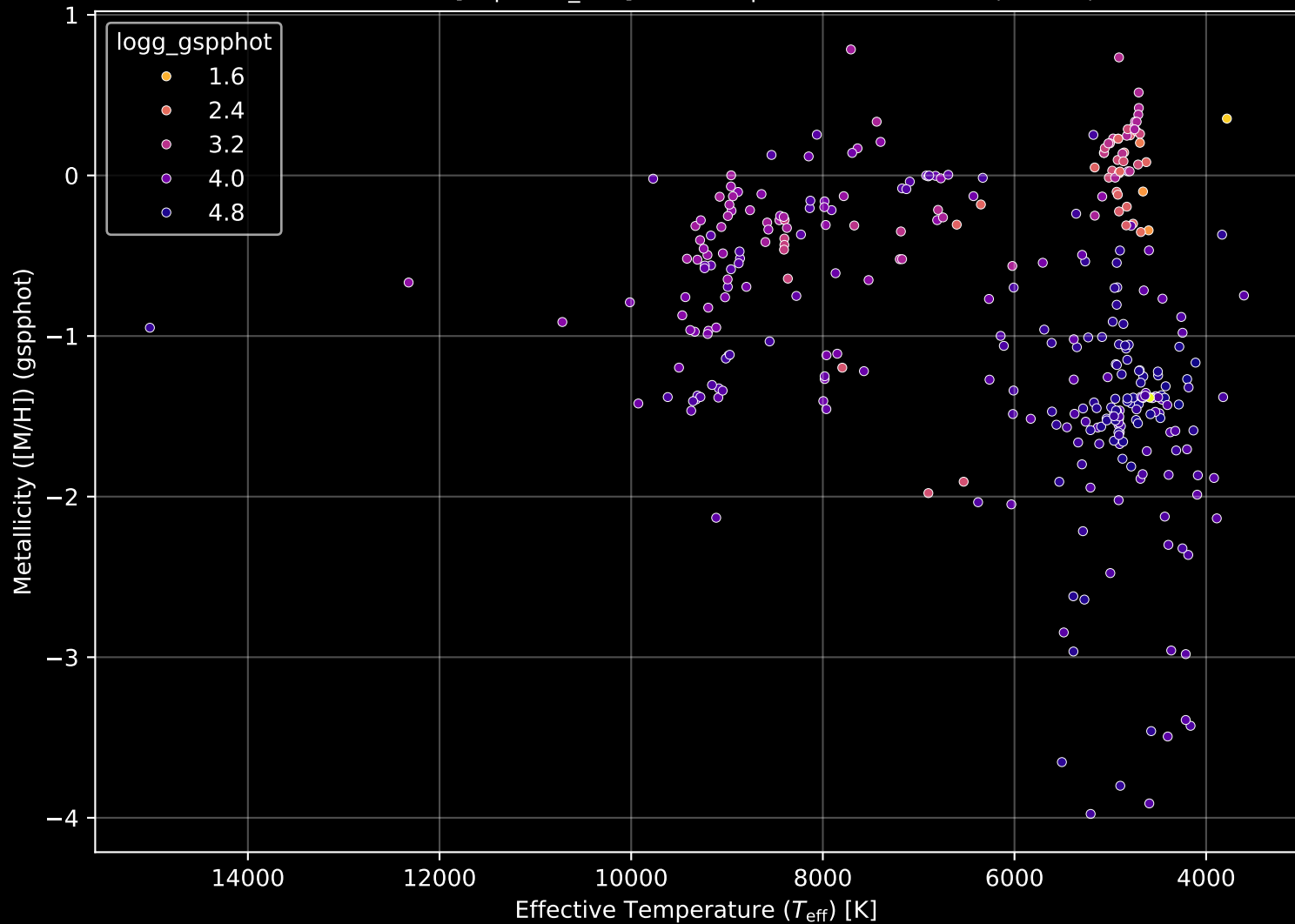
Gaia Cluster: [Ruprecht_143] Stellar Population Parameters (n= 332)
