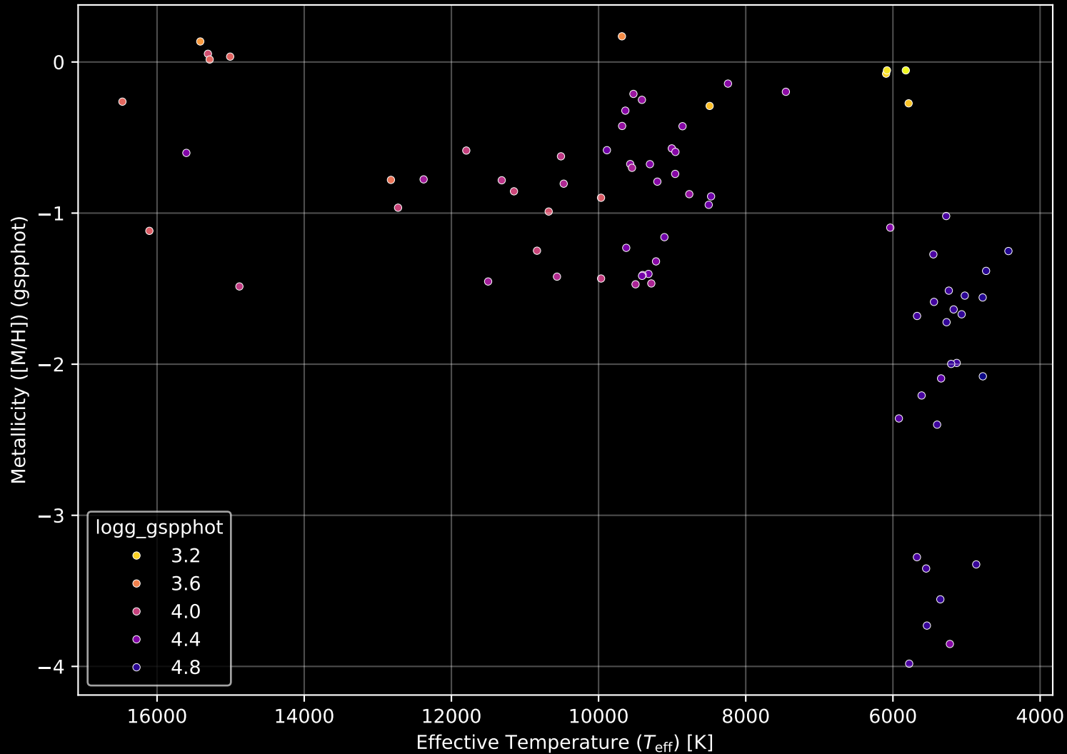
Gaia Cluster: [Ruprecht_148] Stellar Population Parameters (n= 81)
