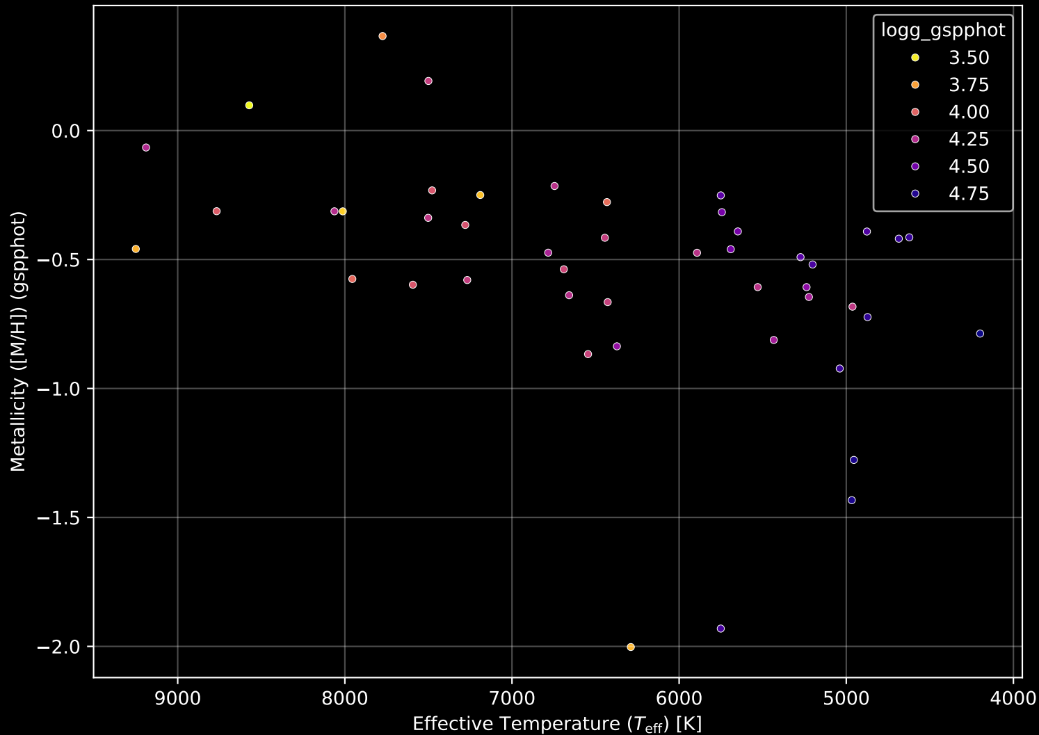
Gaia Cluster: [Ruprecht_151] Stellar Population Parameters (n= 46)
