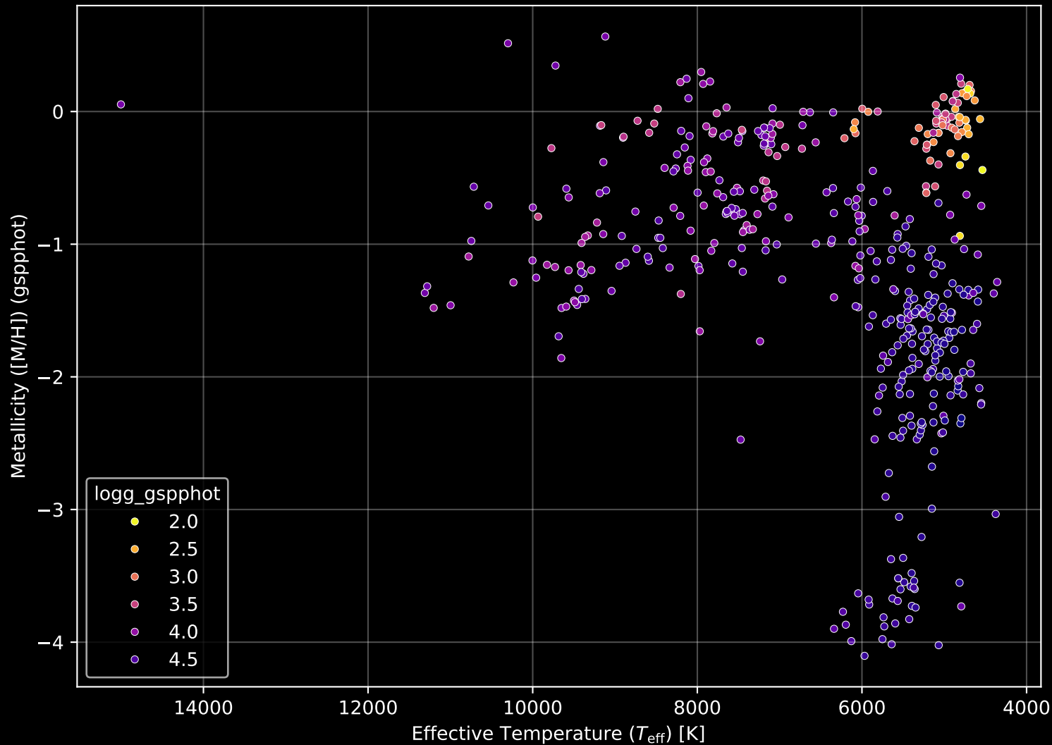
Gaia Cluster: [Ruprecht_164] Stellar Population Parameters (n= 473)
