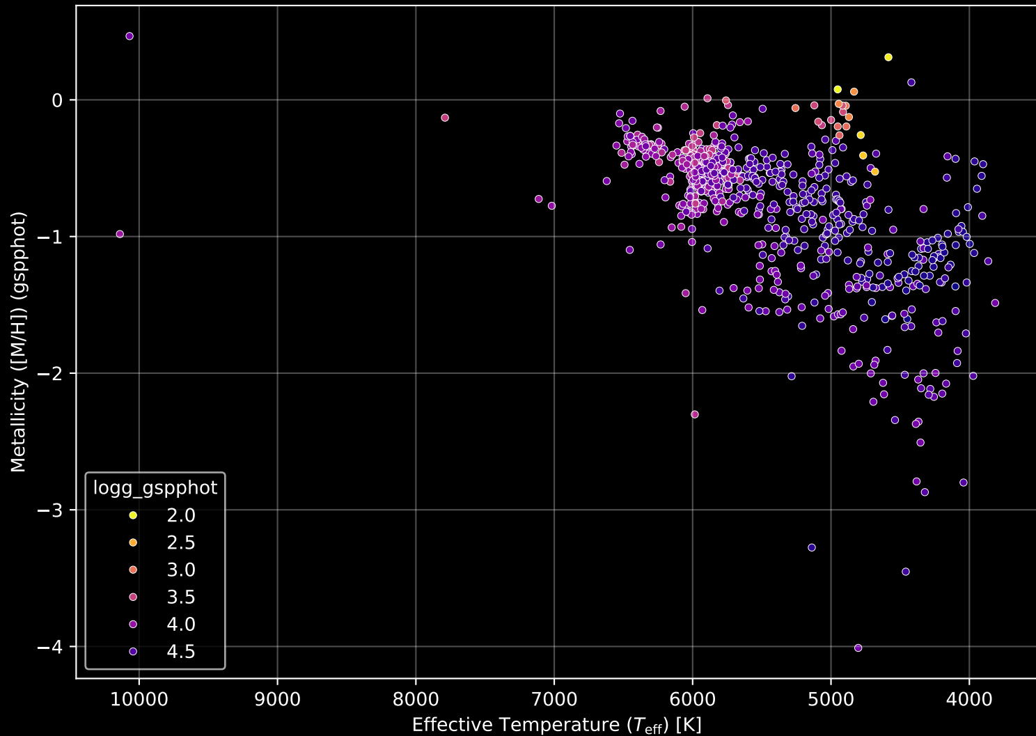
Gaia Cluster: [Ruprecht_171] Stellar Population Parameters (n= 701)
