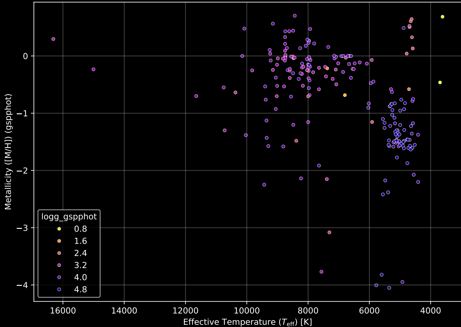
Gaia Cluster: [Ruprecht_176] Stellar Population Parameters (n= 214)
