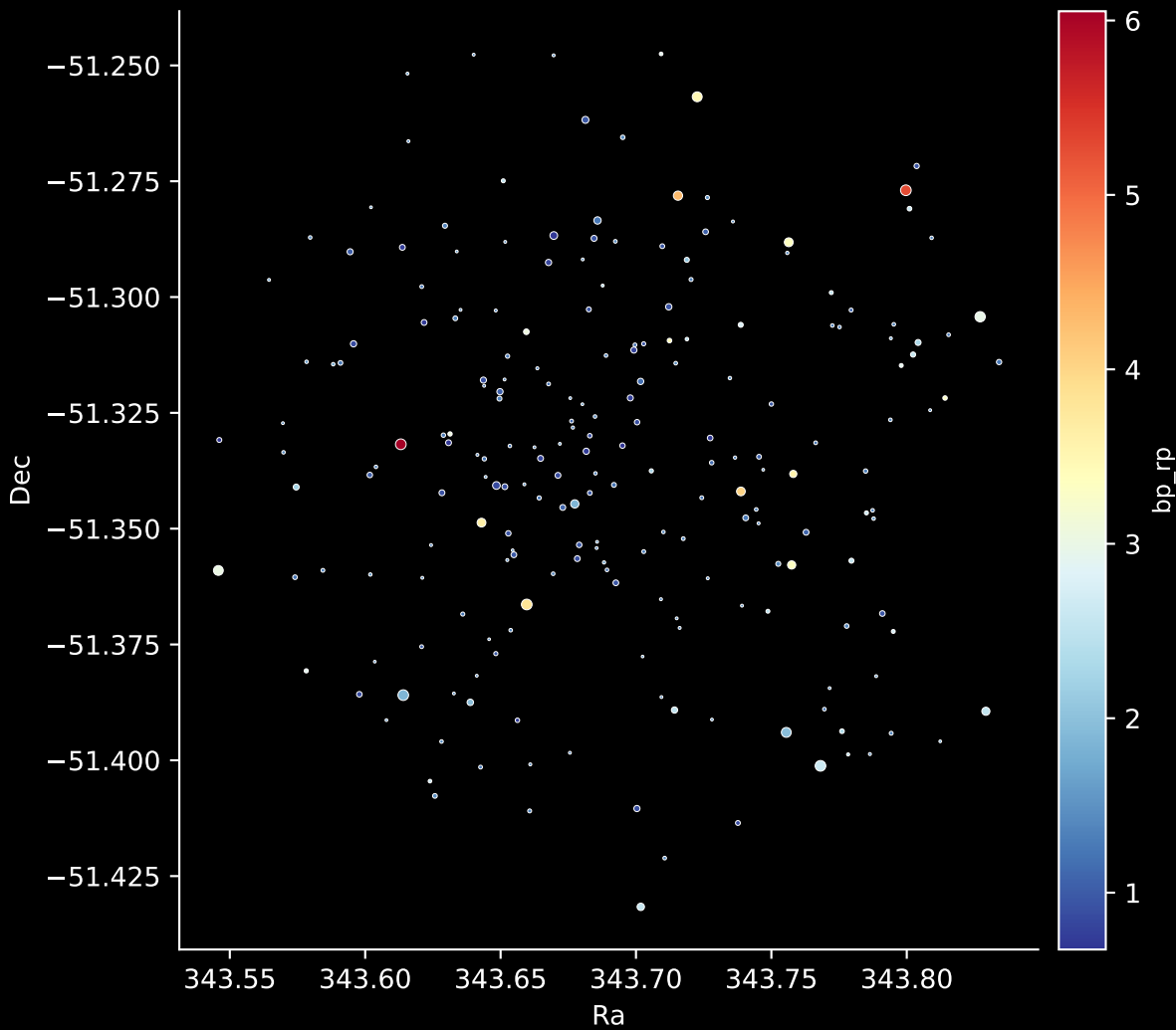
Gaia Cluster: [Ruprecht_176] Stars: 214
