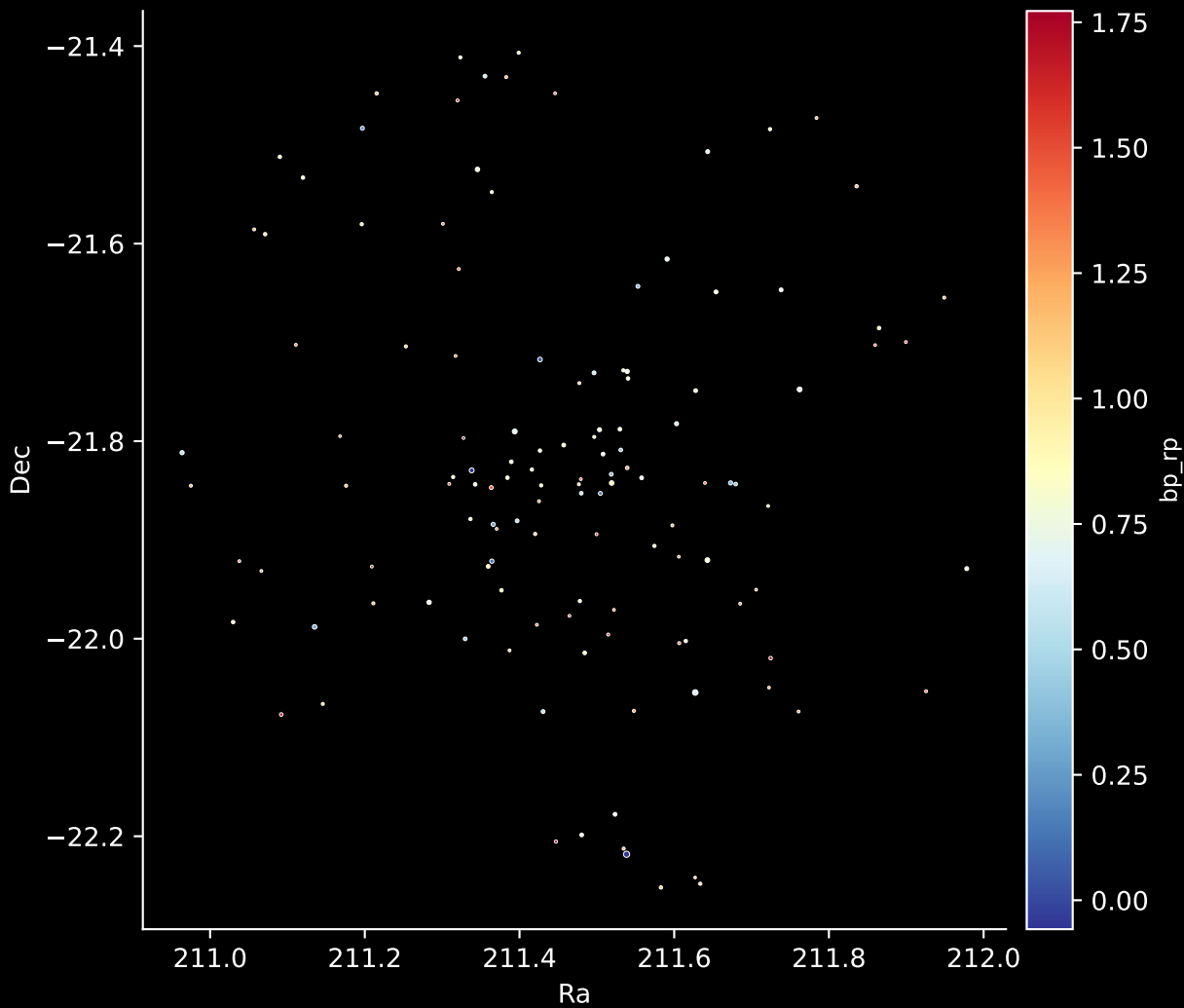
Gaia Cluster: [Ruprecht_19] Stars: 126
