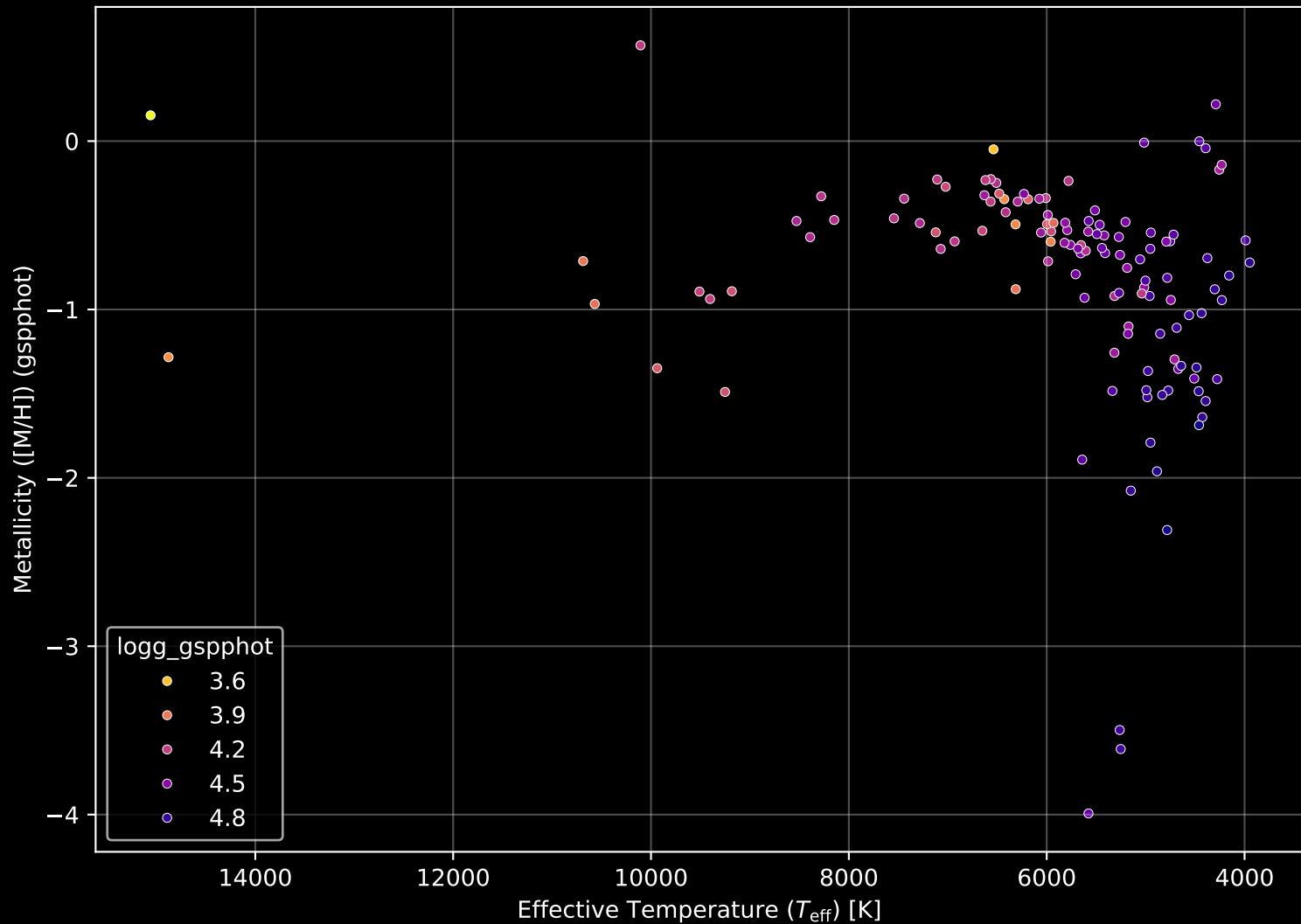
Gaia Cluster: [Ruprecht_19] Stellar Population Parameters (n= 126)
