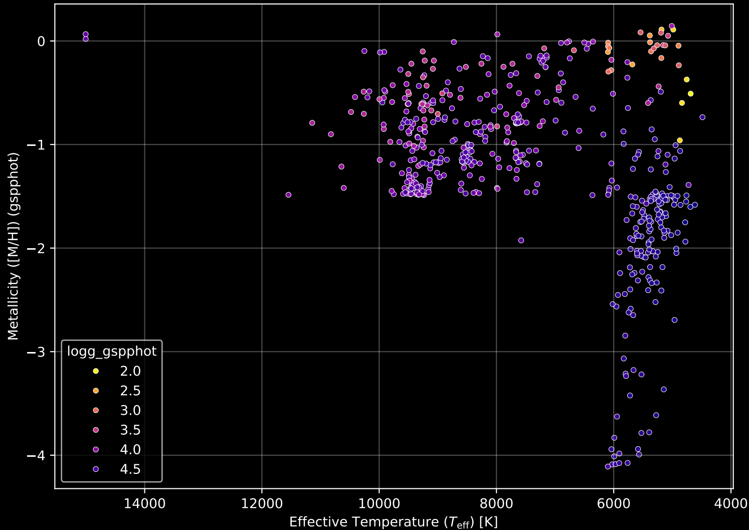
Gaia Cluster: [Ruprecht_23] Stellar Population Parameters (n= 536)
