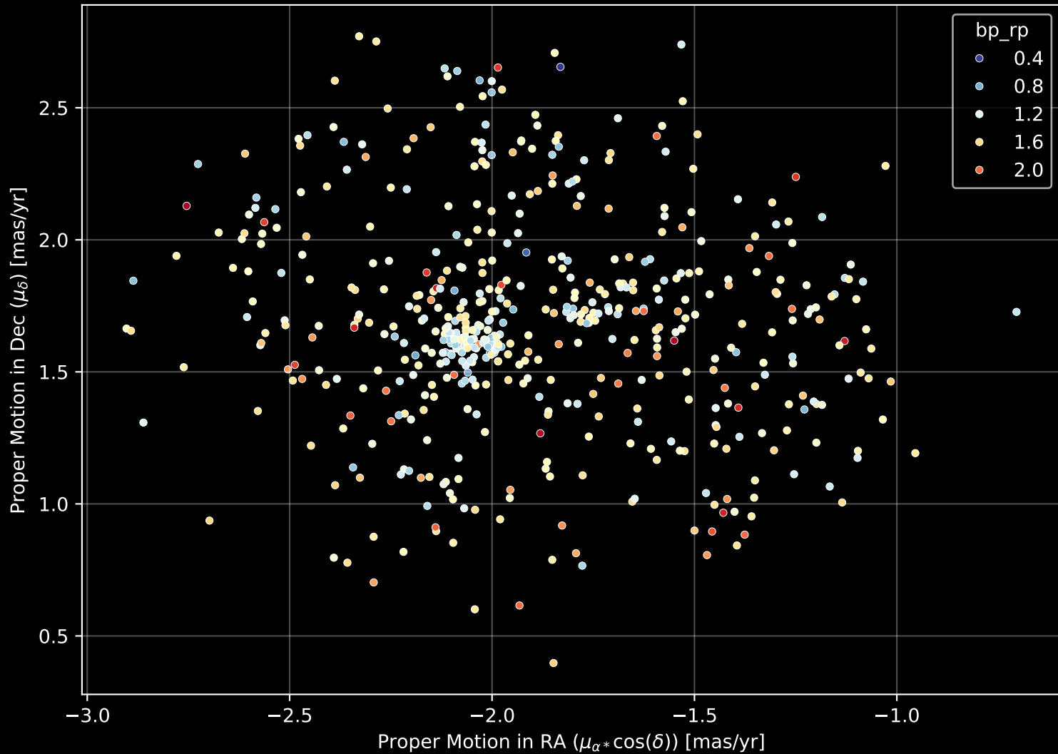
Gaia Cluster: [Ruprecht_23] Proper Motion Diagram (n= 536)
