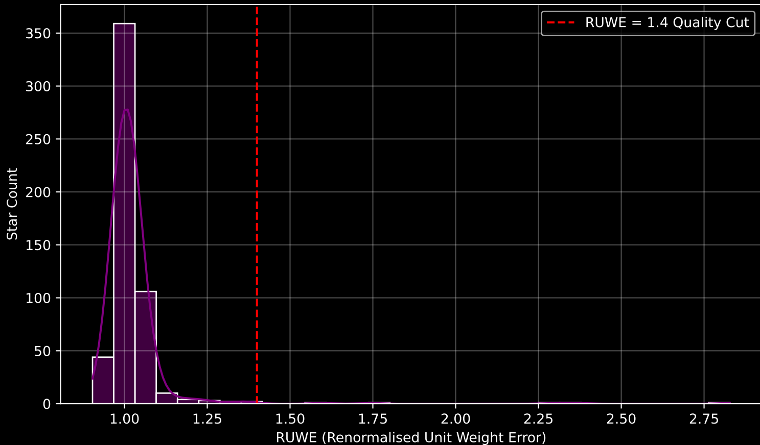
Gaia Cluster: [Ruprecht_23] RUWE Distribution (n= 535)
