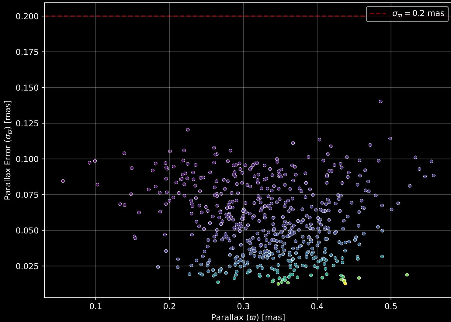
Gaia Cluster: [Ruprecht_23] Parallax Quality (n= 536)
