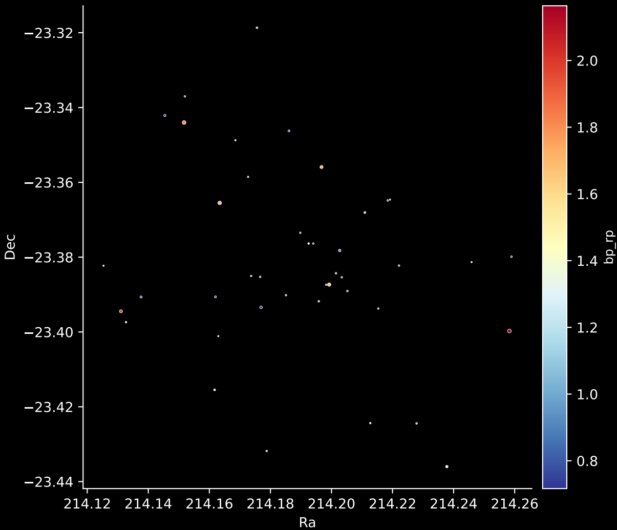
Gaia Cluster: [Ruprecht_25] Stars: 42
