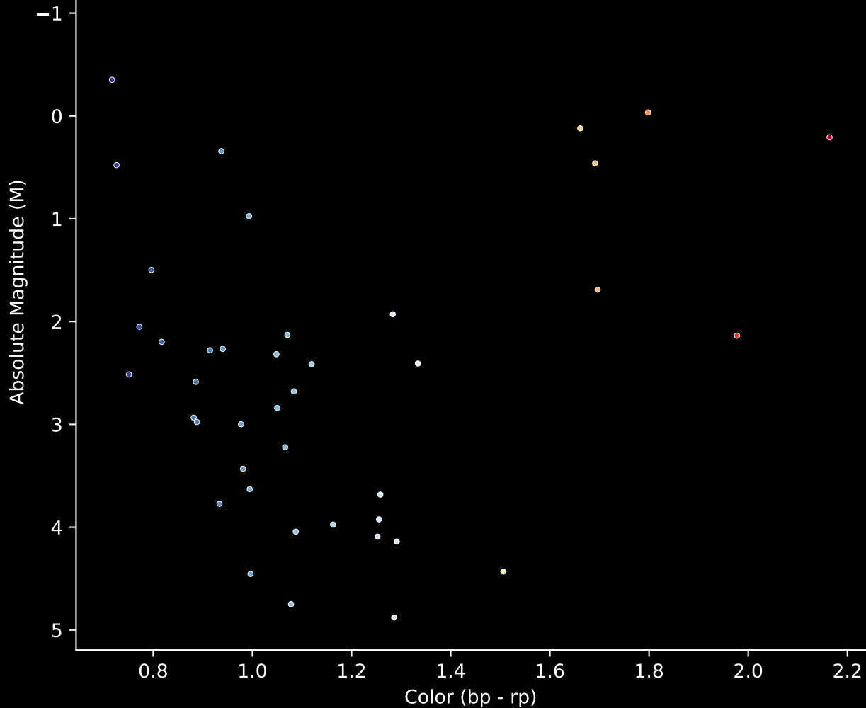
Gaia Cluster: [Ruprecht_25] Stars (n= 42) Hertzsprung-Russel Diagram
