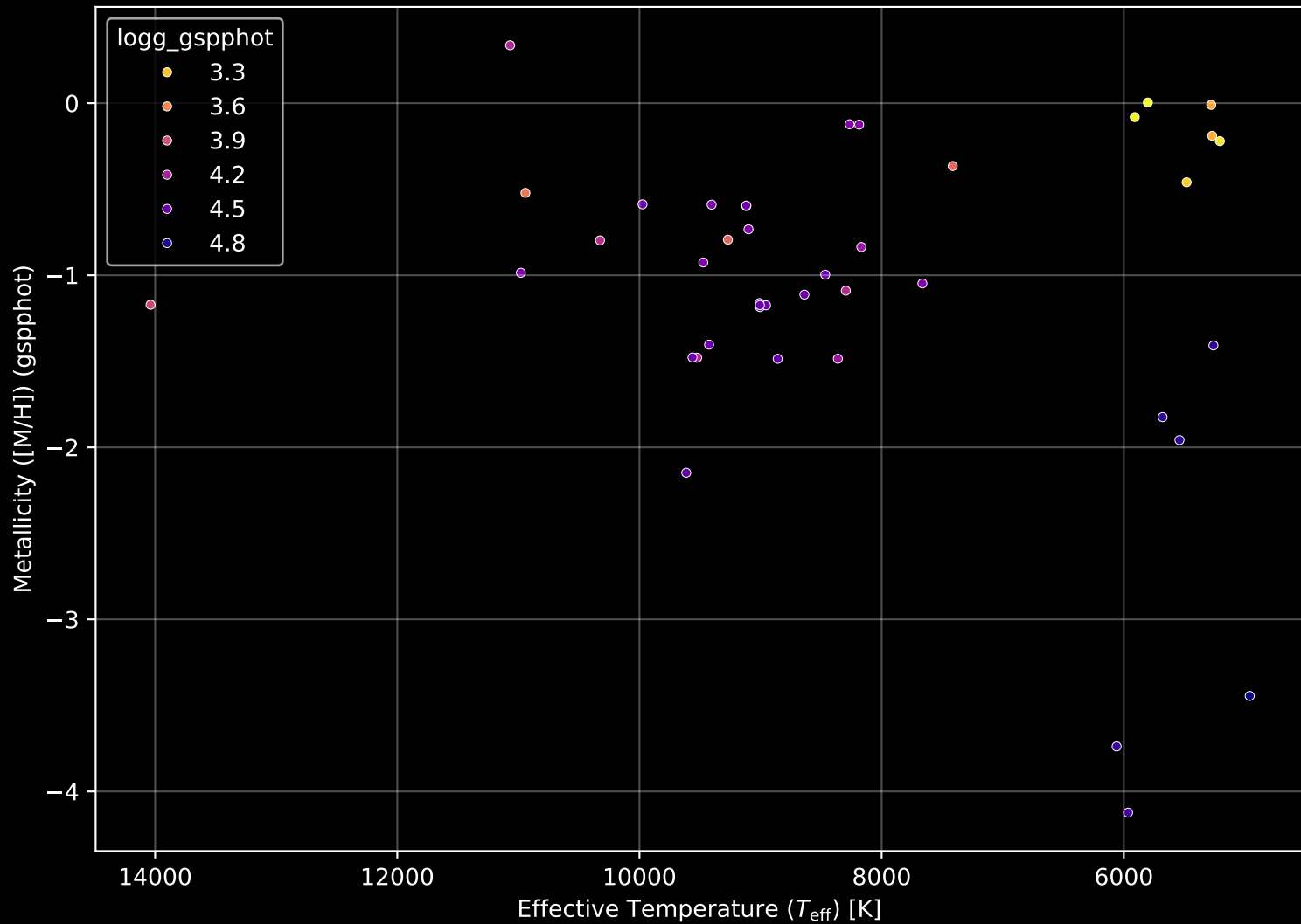
Gaia Cluster: [Ruprecht_25] Stellar Population Parameters (n= 42)
