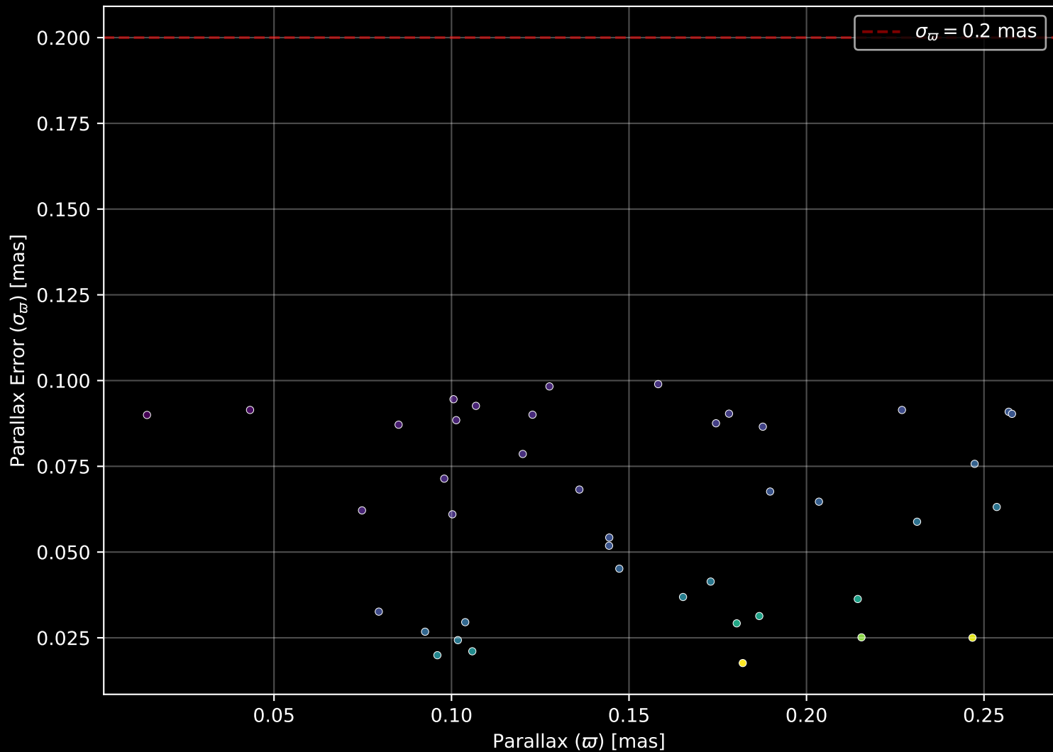
Gaia Cluster: [Ruprecht_25] Parallax Quality (n= 42)
