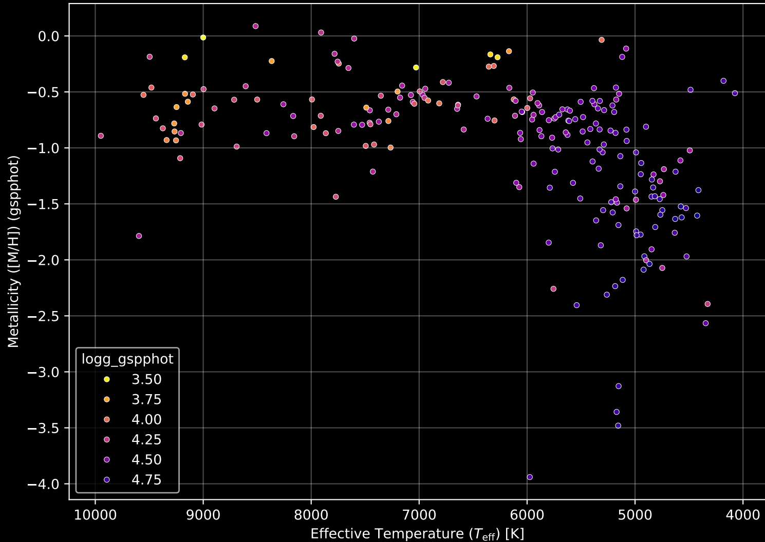
Gaia Cluster: [Ruprecht_27] Stellar Population Parameters (n= 220)
